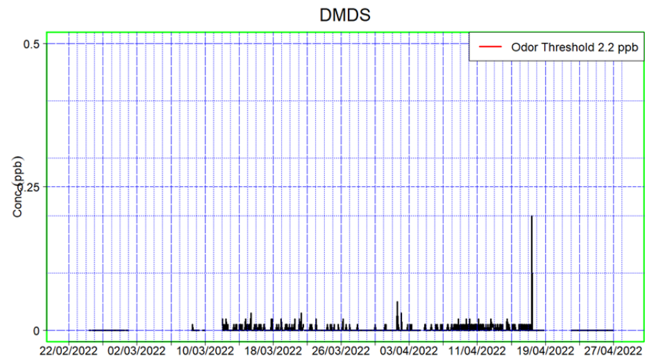
Figura 4: grafici della campagna di misura di Loc. Roncigliano, Albano Laziale (RM) per 2-butil mercaptano, dimetil-solfuro, metil-etil-solfuro, dimetil-disolfuro;
