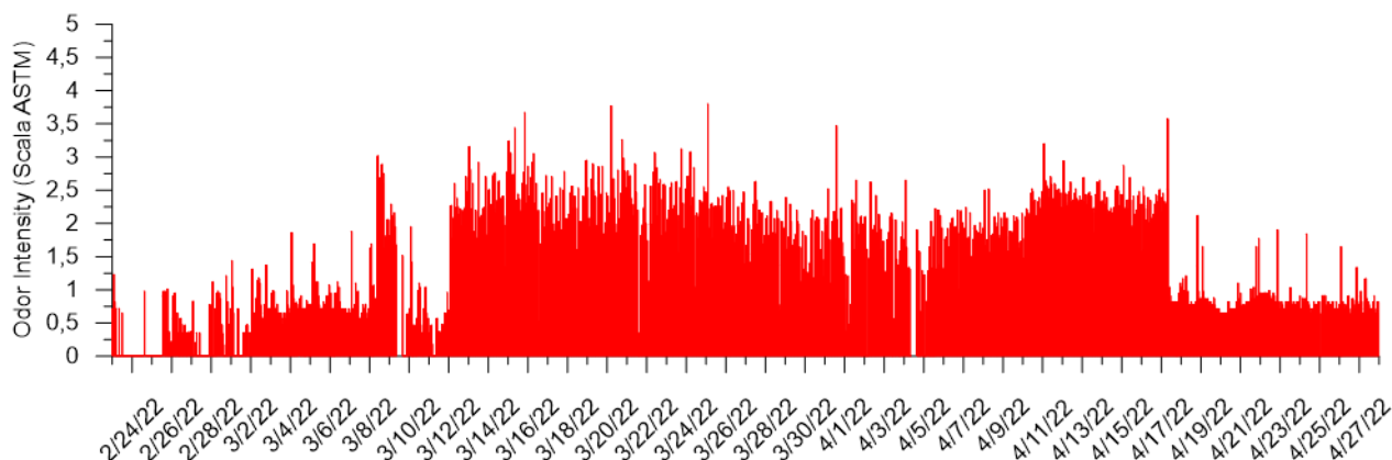
Figura 8 Intensità di odore rilevata durante la campagna di misura
