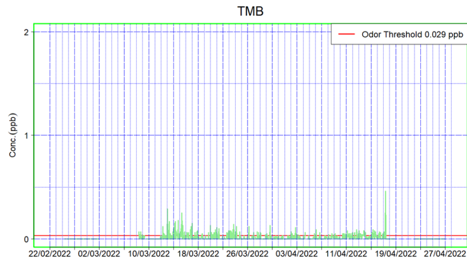
Figura 5: grafici della campagna di misura di Loc. Roncigliano, Albano Laziale (RM) per tetra idro tiofene (THT) e terz-butil-mercaptano (TMB)
