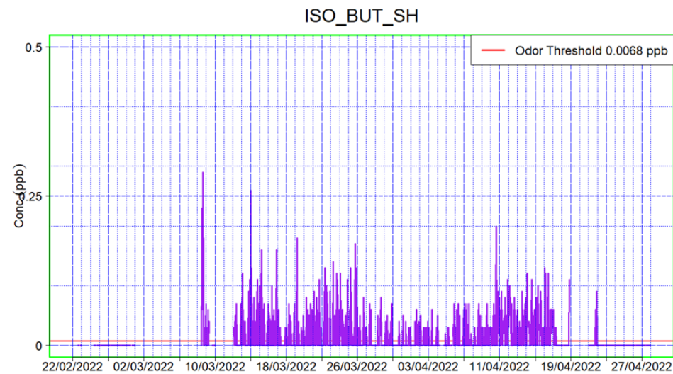
Figura 3: grafici della campagna di misura a Loc. Roncigliano, Albano Laziale (RM) per N-propil-mercaptano, iso-propil-mercaptano, N-butil-mercaptano, iso-butil-mercaptano;
