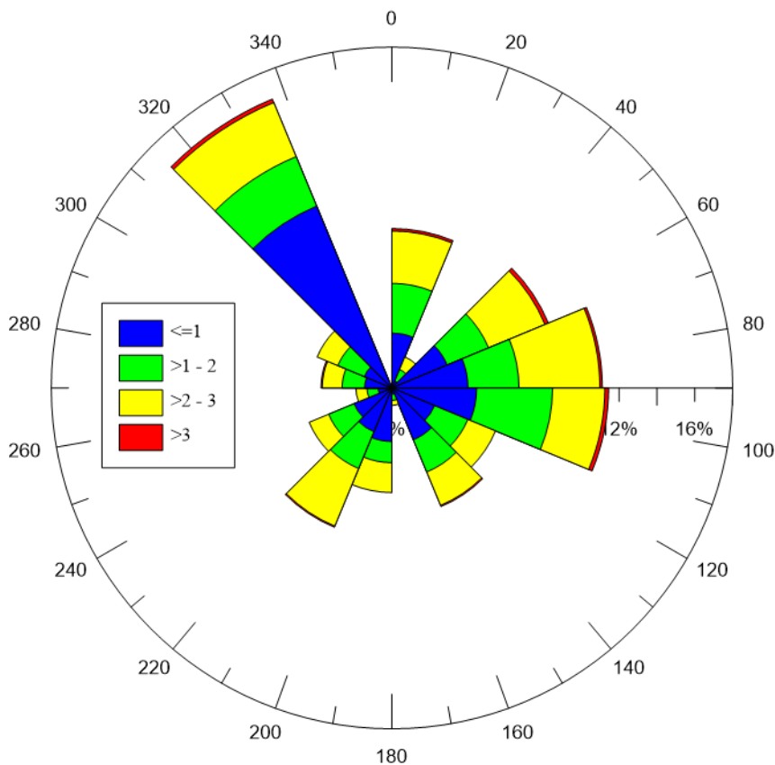
Figura 9 Intensità di odore in funzione della direzione del vento prevalente su base oraria.
