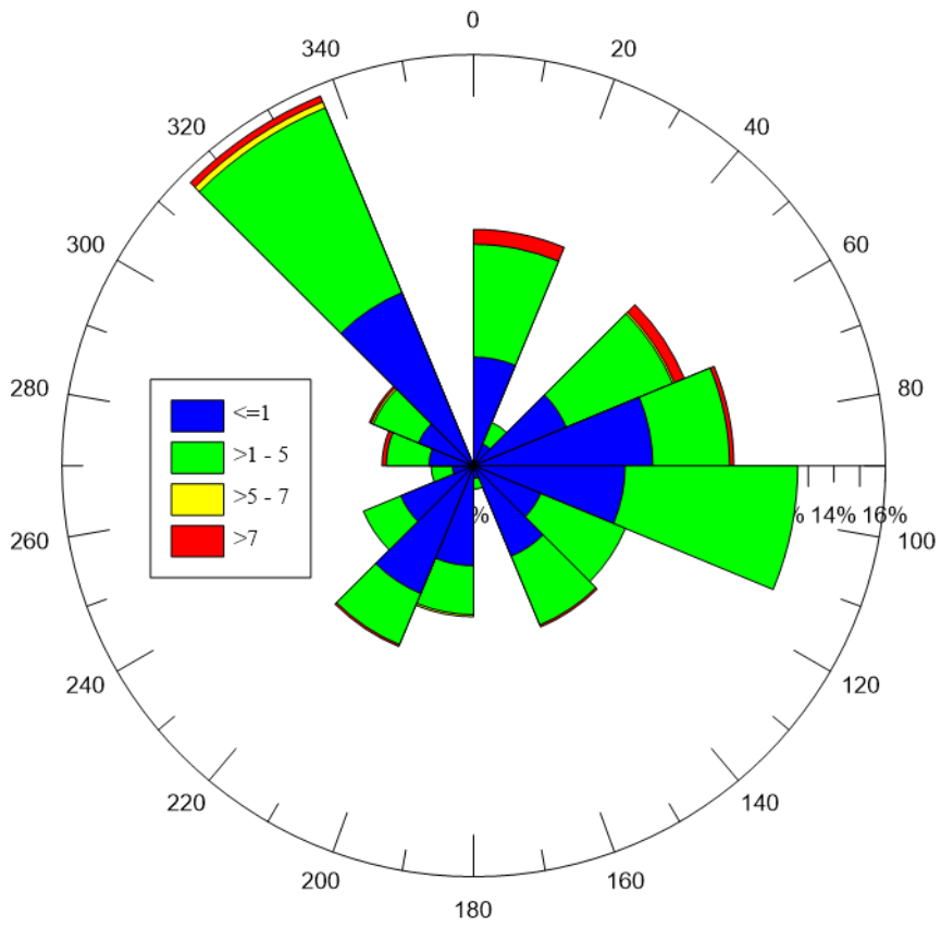
Figura 11: rosa delle concentrazioni di picco dell'H 2 S
