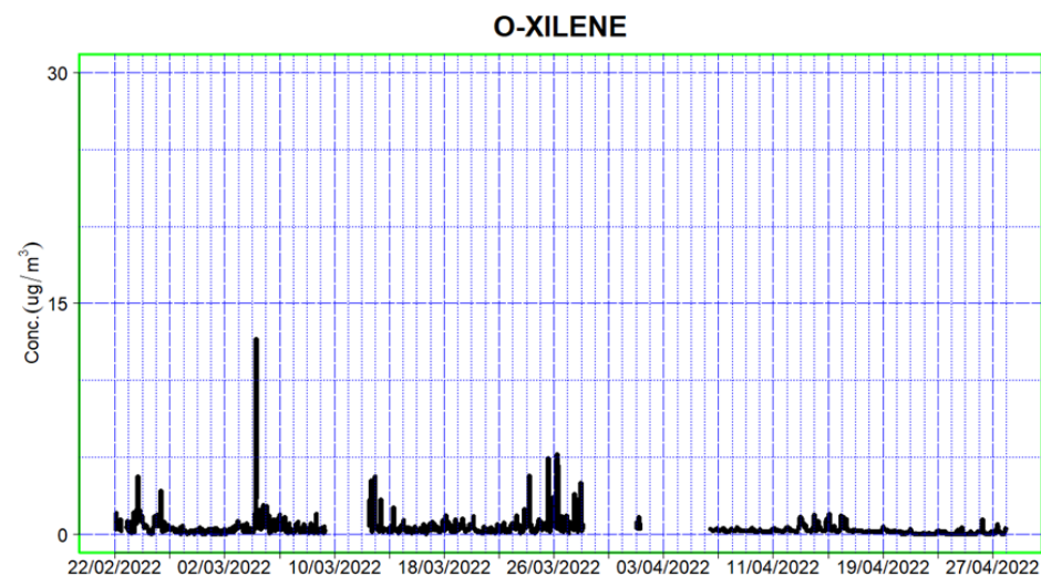
Figura 6: grafici della campagna di misura di Loc. Roncigliano, Albano Laziale (RM) per benzene, toluene, MP-xilene, o-xilene.
