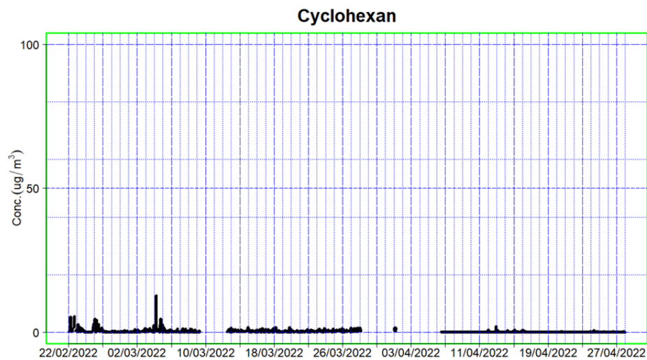
Figura 7: grafici della campagna di misura di Loc. Roncigliano, Albano Laziale (RM) per etilbenzene, styrene, ciclohexan
