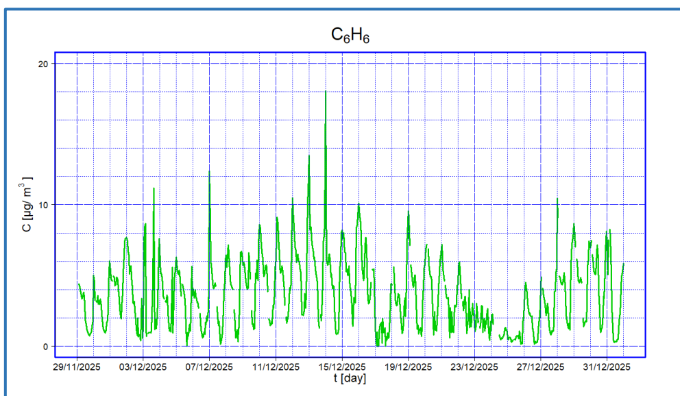
Figura 13 - Valori medi orari di concentrazione di C_6H_6 – II periodo
