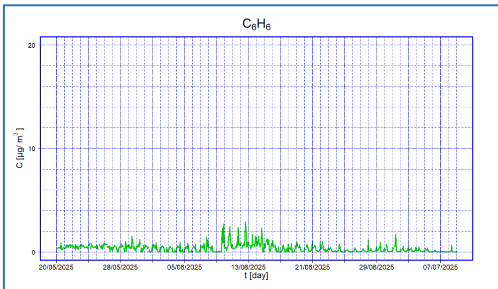
Figura 12 - Valori medi orari di concentrazione di C_6H_6 – I periodo
