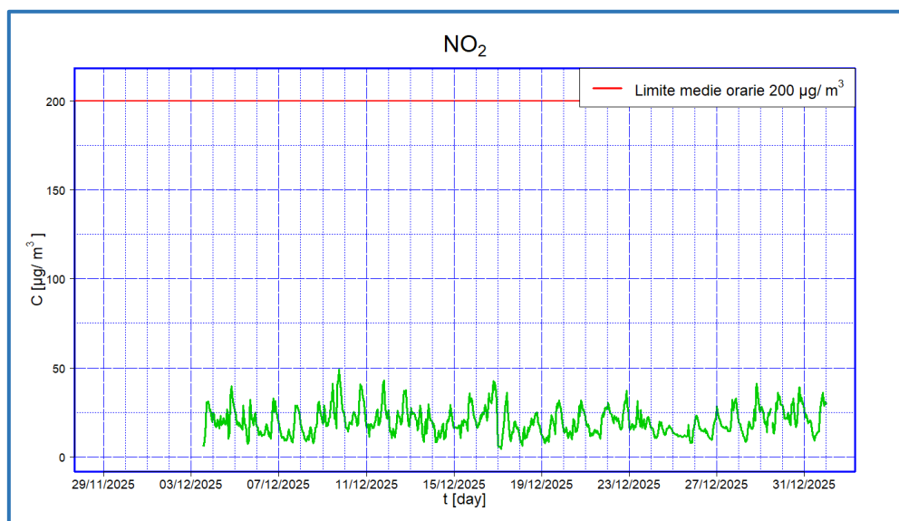
Figura 11 - Valori medi orari di concentrazione di \text{NO}_2 – II periodo
