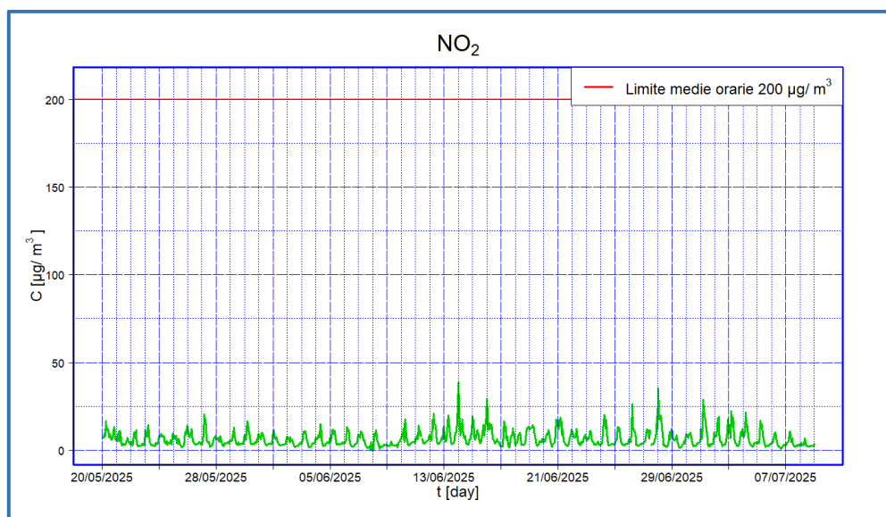
Figura 10 - Valori medi orari di concentrazione di \text{NO}_2 – I periodo
