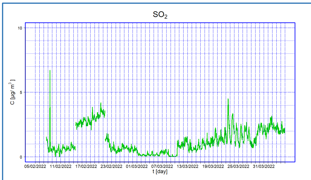
Figura 13 - Valori medi orari di concentrazione di SO_2 - periodo I campagna
