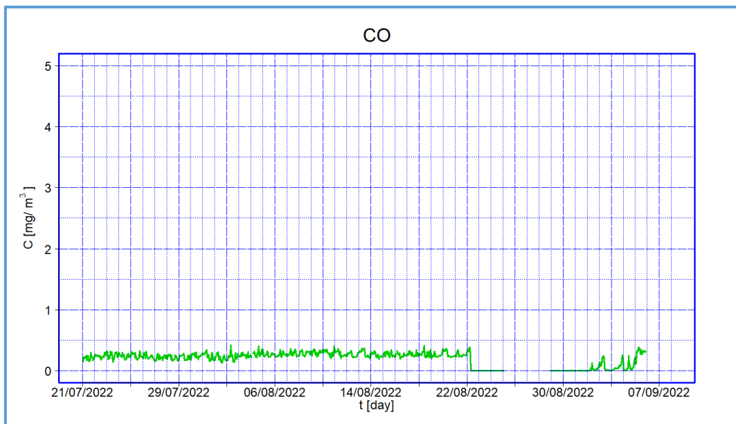
Figura 16 - Valori medi orari di concentrazione di CO - periodo II campagna
