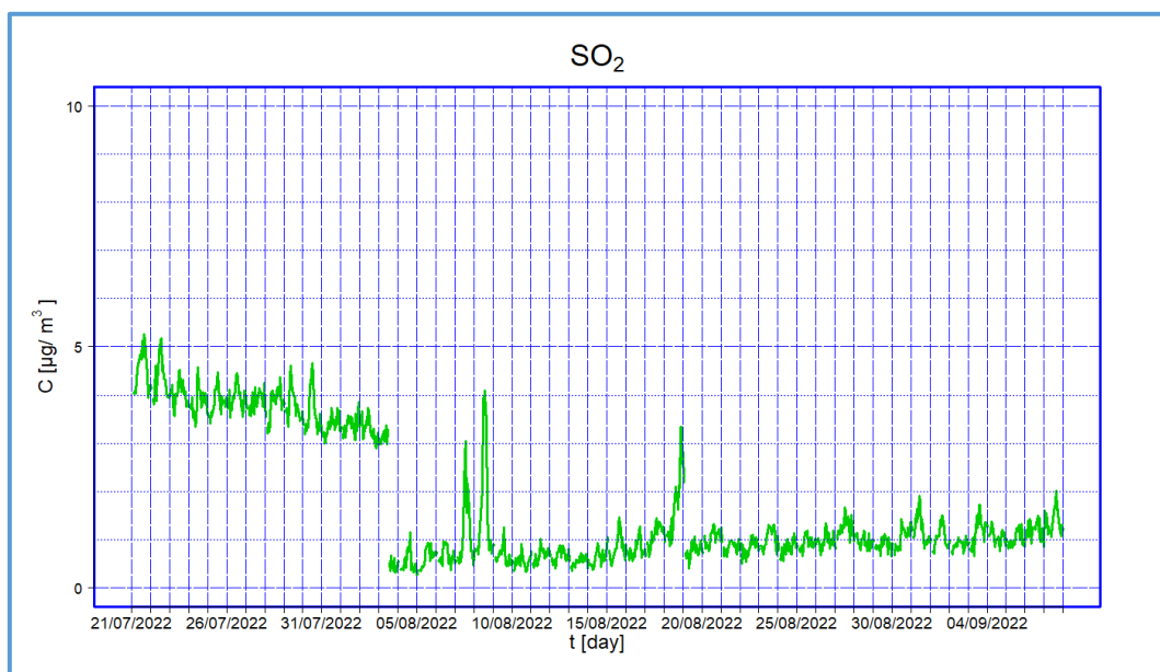
Figura 14 - Valori medi orari di concentrazione di SO_2 - periodo II campagna
