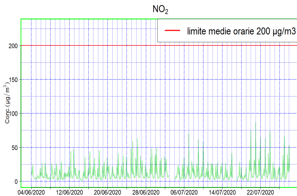
Figura 5: Valori orari di NO 2
