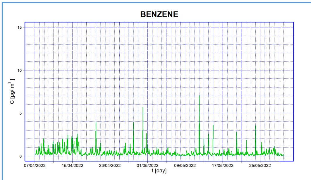
Figura 18 - Valori medi orari di concentrazione di C_6H_6 - periodo I campagna
