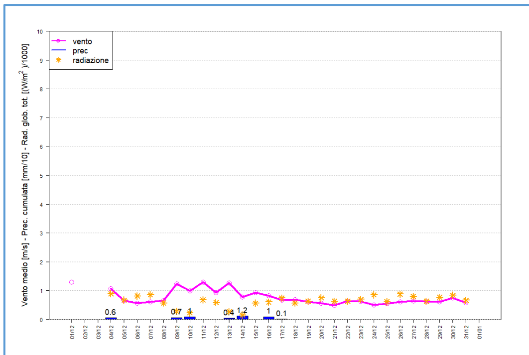
Figura 5 - Vento medio, Precipitazione cumulata e Radiazione Globale Totale
