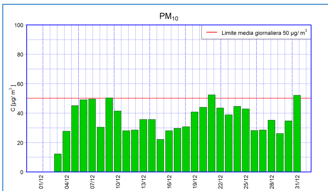
Figura 9 - Valori giornalieri di concentrazione di PM10 - periodo II campagna
