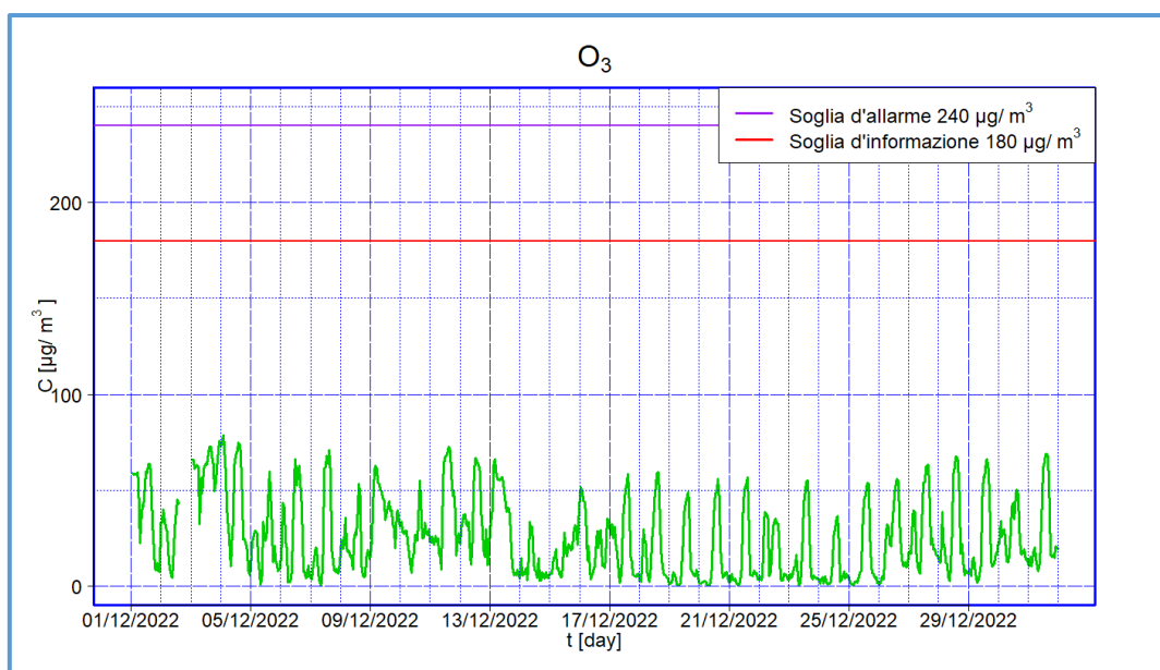
Figura 15 - Valori medi orari di concentrazione di O 3 - periodo II campagna
