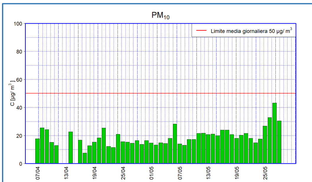
Figura 8 - Valori giornalieri di concentrazione di PM10 - periodo I campagna
