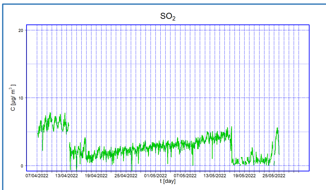
Figura 16 - Valori medi orari di concentrazione di SO_2 - periodo I campagna
