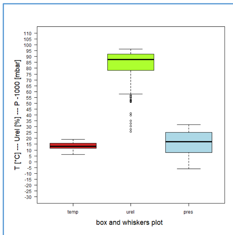
Figura 7 - Temperatura, Umidità relativa e Pressione
