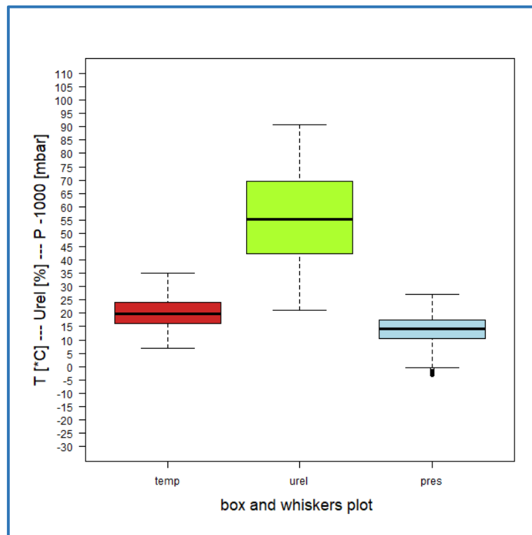
Figura 4 - Temperatura, Umidità relativa e Pressione
