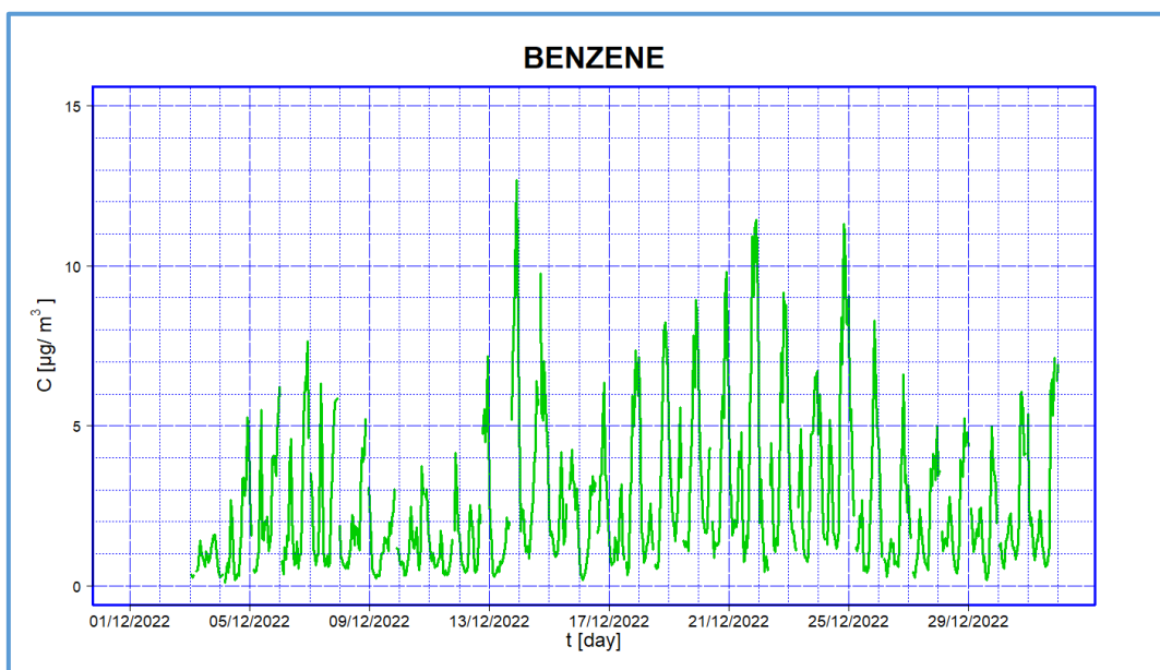
Figura 19 - Valori medi orari di concentrazione di C_6H_6 - periodo II campagna
