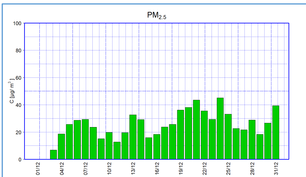
Figura 11 - Valori giornalieri di concentrazione di PM2.5 - periodo II campagna
