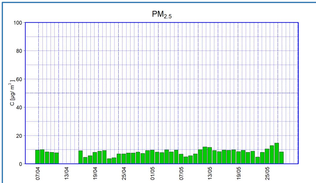
Figura 10 - Valori giornalieri di concentrazione di PM2.5 - periodo I campagna
