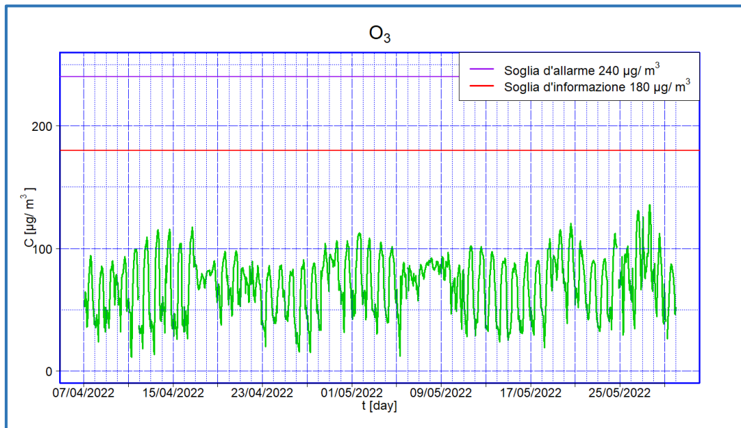
Figura 14 - Valori medi orari di concentrazione di O 3 - periodo I campagna
