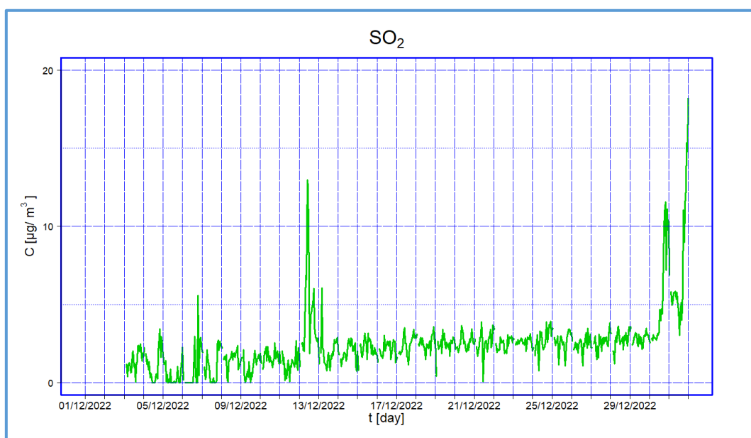
Figura 17 - Valori medi orari di concentrazione di SO_2 - periodo II campagna
