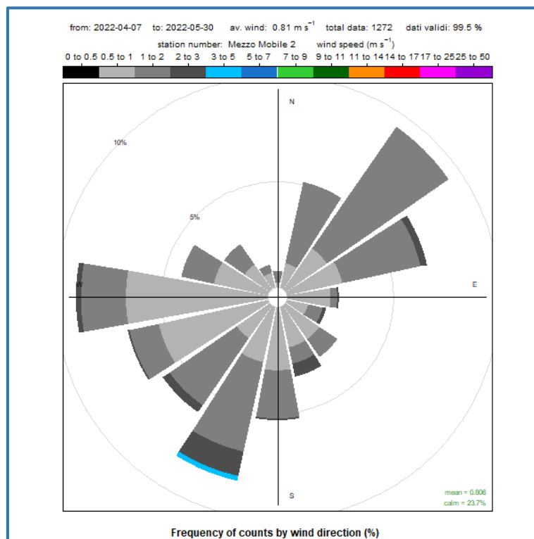
Figura 3 - Rosa dei venti
