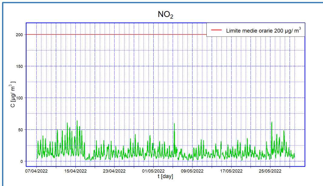
Figura 12 - Valori medi orari di concentrazione di \text{NO}_2 - periodo I campagna
