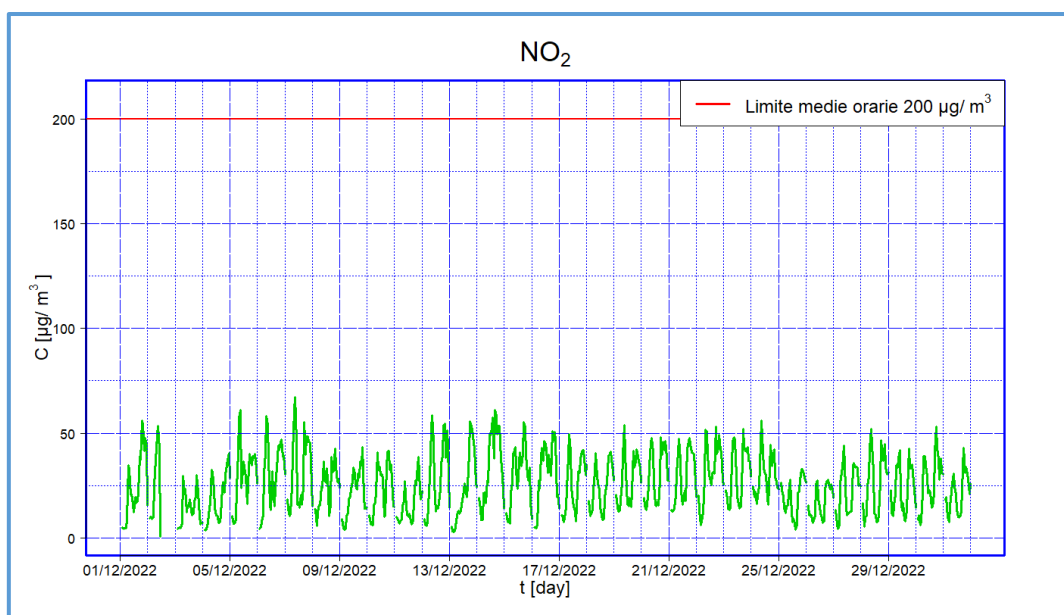
Figura 13 - Valori medi orari di concentrazione di \text{NO}_2 - periodo II campagna
