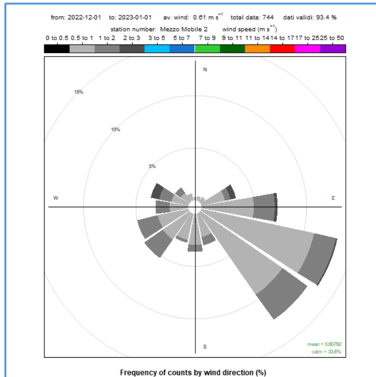
Figura 6 - Rosa dei venti
