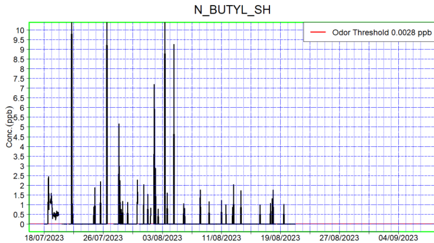
Figura 3: grafici della campagna di misura presso Gallese per N-propil-mercaptano, iso-propil-mercaptano, N-butil-mercaptano e iso-butil-mercaptano;
