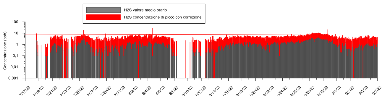
Figura 8 Concentrazione media (grigio) e di picco (rosso) dell'H 2 S rilevata durante la campagna di misura. Nel grafico è riportato il valore di 7 µg/m 3 , sotto il quale secondo l'OMS dovrebbero rimanere le concentrazioni medie semiorarie di questo inquinante per non arrecare molestia olfattiva.
