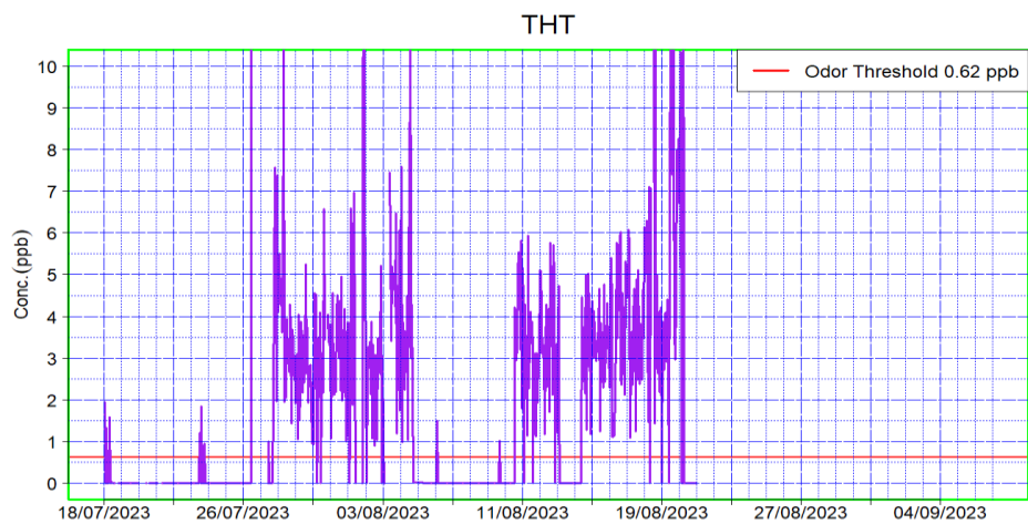
Figura 5: grafici della campagna di misura presso Gallese per tetra idro tiofene (THT) e terz-butyl-mercaptano (TMB)
