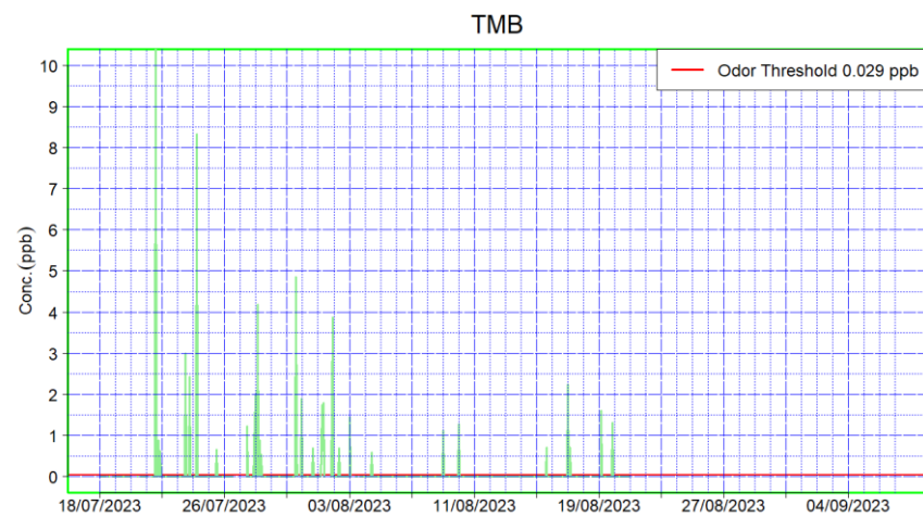
Figura 5: grafici della campagna di misura presso Gallese per tetra idro tiofene (THT) e terz-butyl-mercaptano (TMB)
