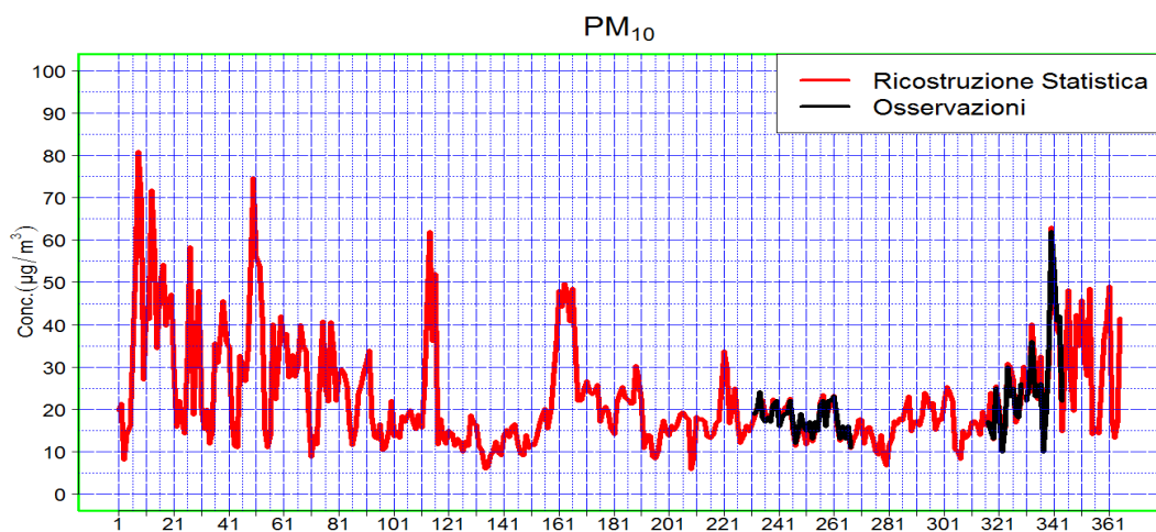
Figura 14: Valori di PM 10 ( \mu\text{g}/\text{m}^3 ) ricostruiti nel 2019 in rosso, mentre in nero i valori osservati
