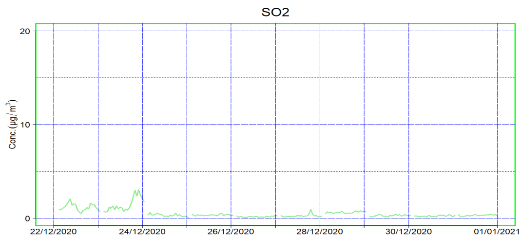
Figura 11: Valori orari di SO 2 nel periodo suddetto (II° campagna)
