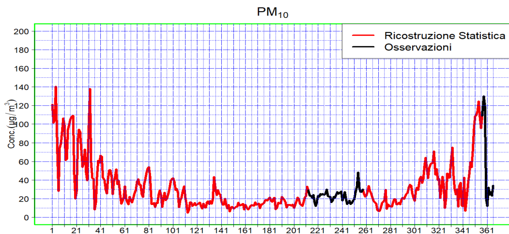
Figura 14: Valori di PM10 ( \mu\text{g}/\text{m}^3 ) ricostruiti nel 2020 in rosso, mentre in nero i valori osservati
