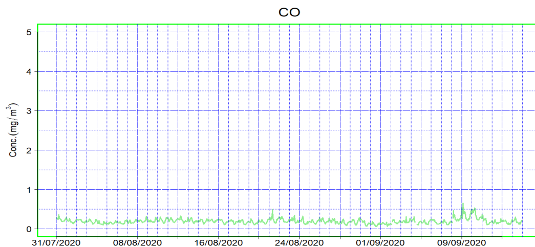
Figura 12: Valori orari di CO nel periodo suddetto (1° campagna)
