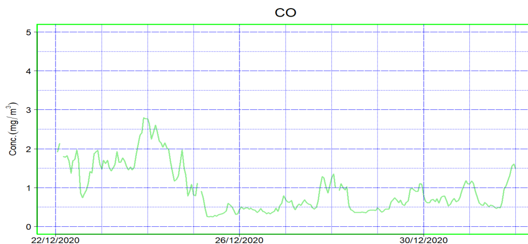
Figura 13: Valori orari di CO nel periodo suddetto (2° campagna)
