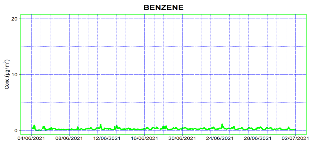
Figura 12: Valori orari di Benzene nel periodo suddetto (II° campagna)
