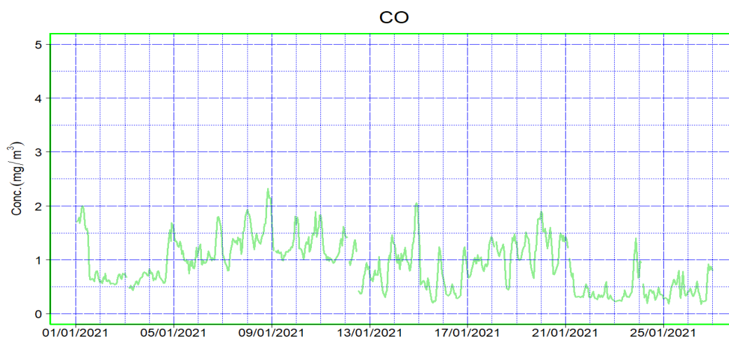
Figura 13: Valori orari di CO nel periodo suddetto (1° campagna)
