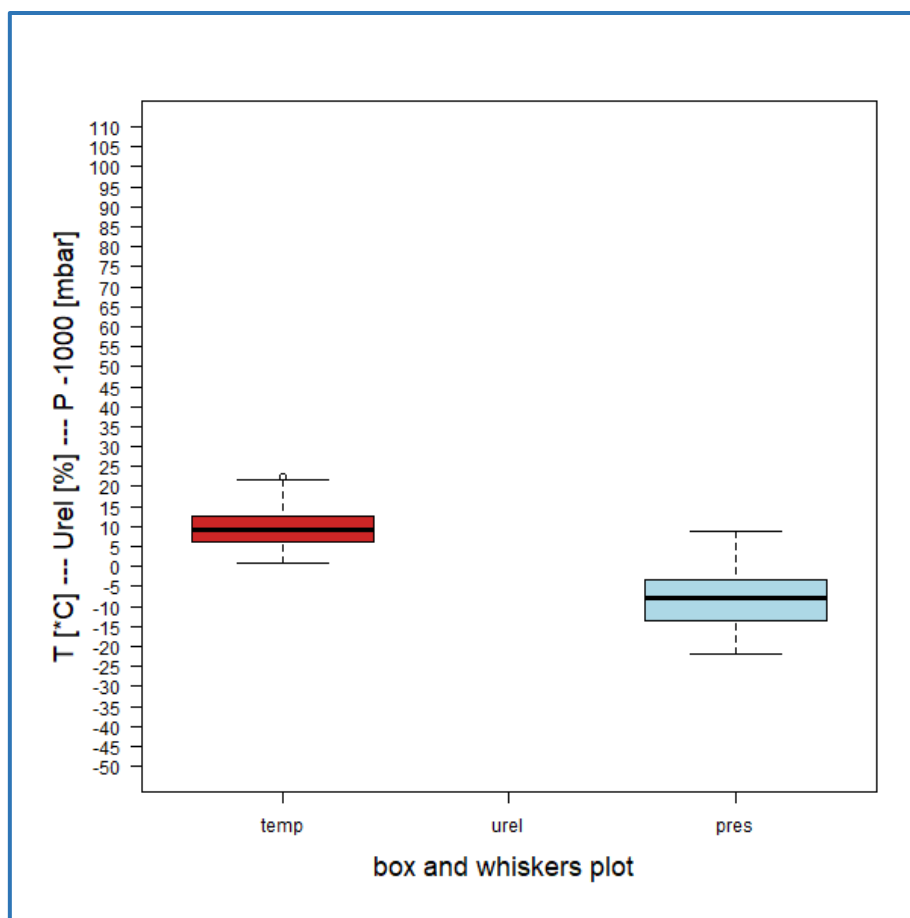
Figura 7 - Temperatura, Umidità relativa e Pressione – II periodo
