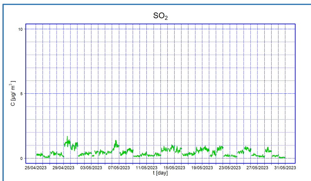
Figura 16 - Valori medi orari di concentrazione di SO_2 – I periodo
