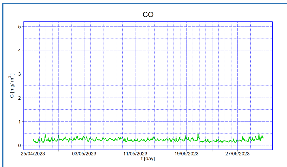
Figura 18 - Valori medi orari di concentrazione di CO – I periodo
