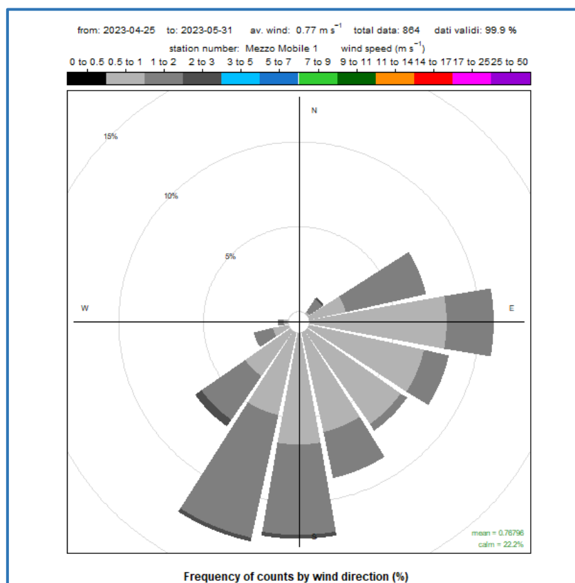
Figura 3 - Rosa dei venti – I periodo
