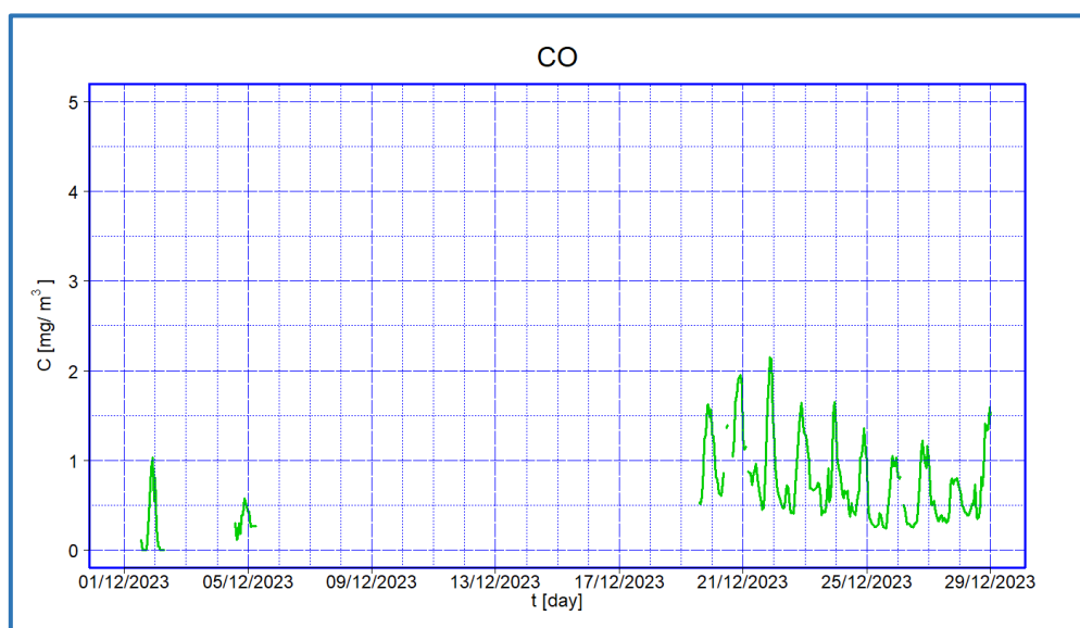
Figura 19 - Valori medi orari di concentrazione di CO – II periodo
