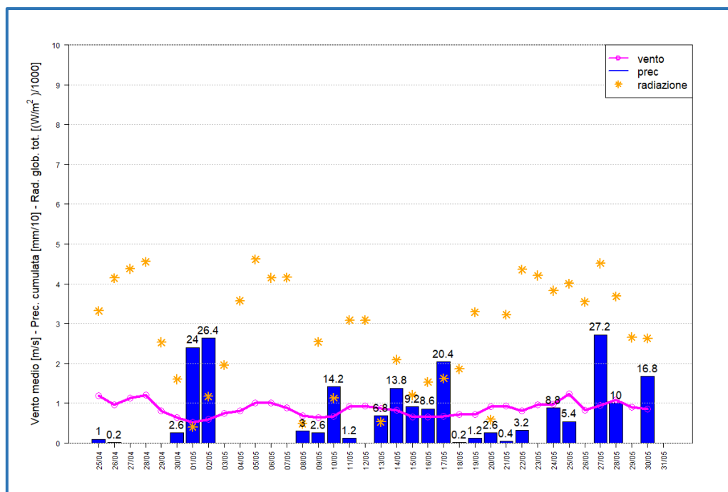
Figura 2 - Vento medio, Precipitazione cumulata e Radiazione Globale Totale – I periodo
