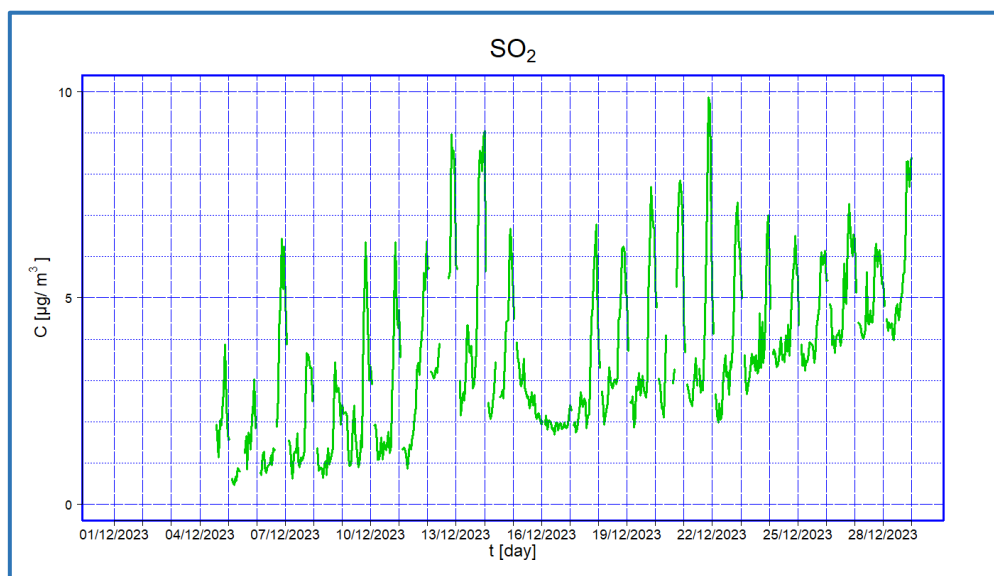
Figura 17 - Valori medi orari di concentrazione di SO_2 – II periodo
