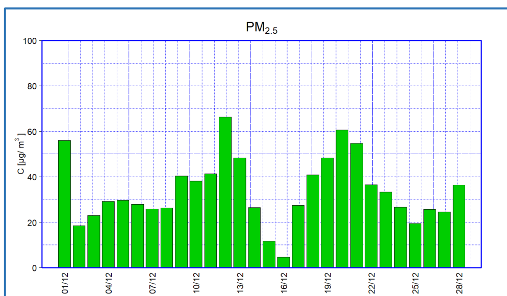
Figura 11 - Valori giornalieri di concentrazione di PM 2.5 – II periodo
