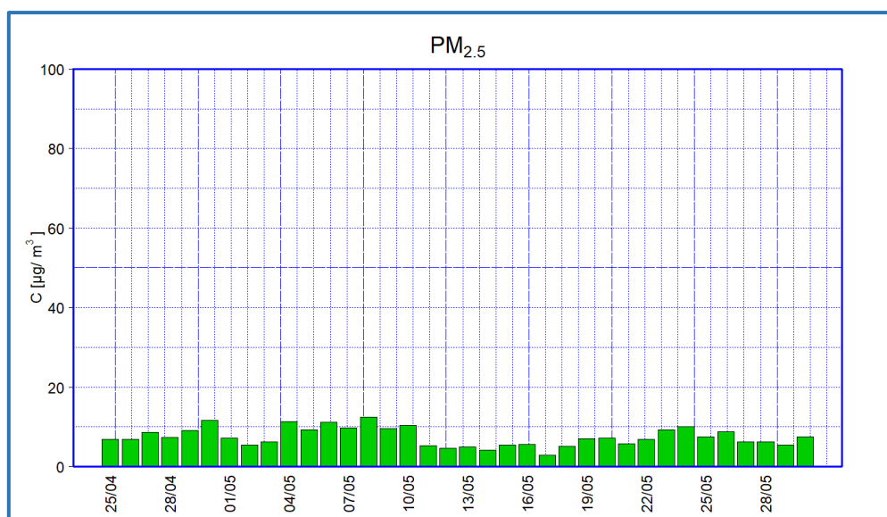
Figura 10 - Valori giornalieri di concentrazione di PM 2.5 – I periodo
