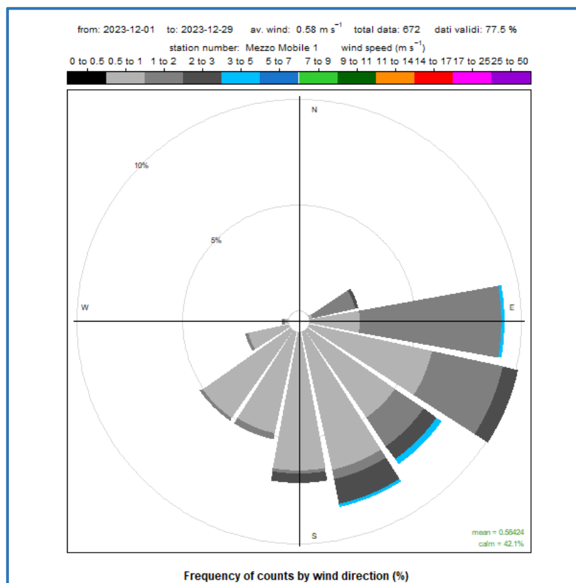
Figura 6 - Rosa dei venti – II periodo
