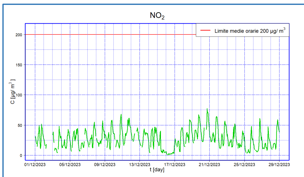
Figura 13 - Valori medi orari di concentrazione di \text{NO}_2 – II periodo
