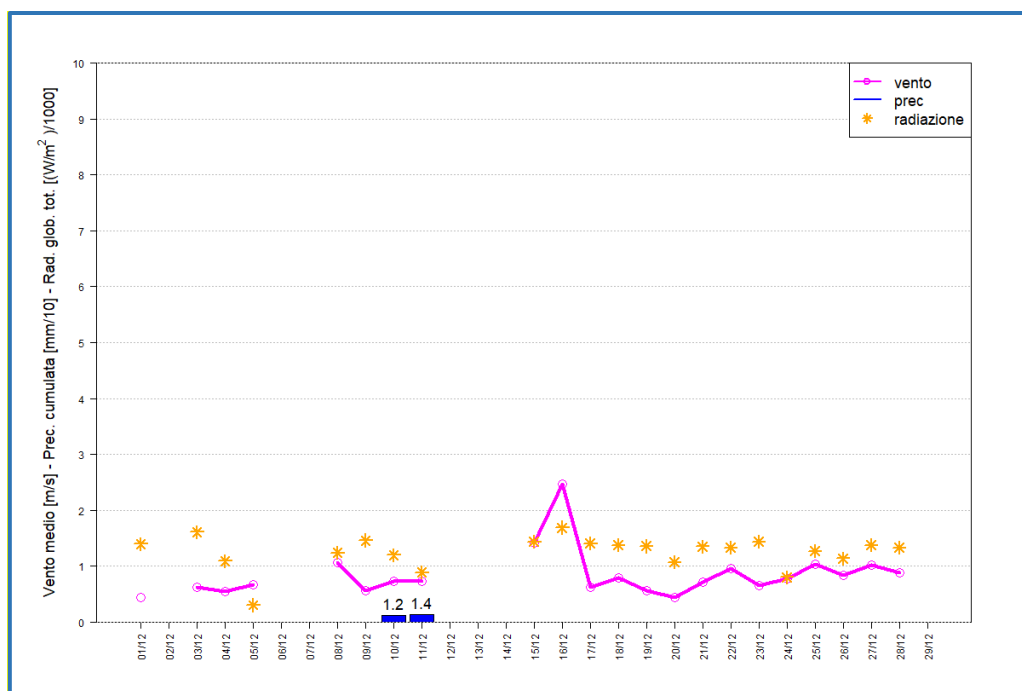
Figura 5 - Vento medio, Precipitazione cumulata e Radiazione Globale Totale – II periodo
