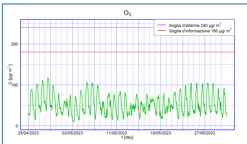
Figura 14 - Valori medi orari di concentrazione di O_3 - I periodo
