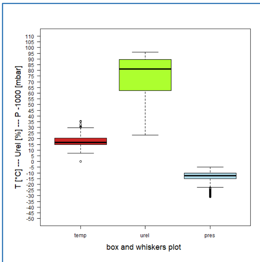
Figura 4 - Temperatura, Umidità relativa e Pressione – I periodo
