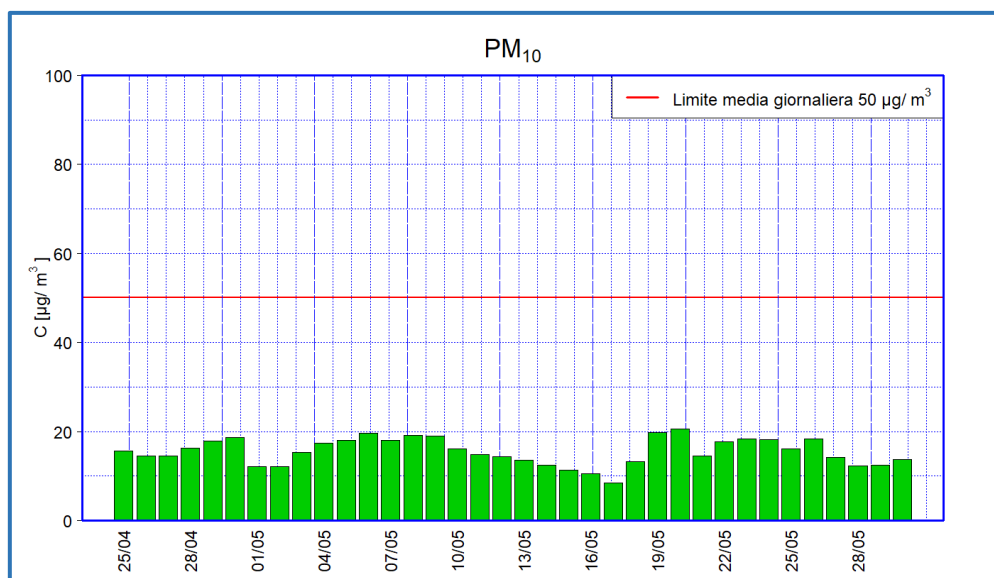
Figura 8 - Valori giornalieri di concentrazione di PM 10 – I periodo
