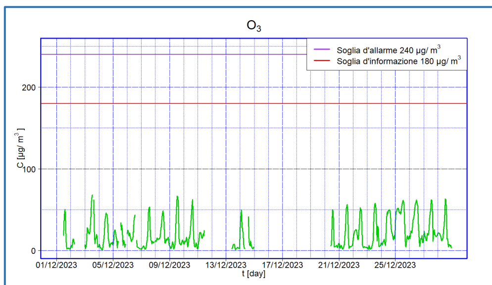
Figura 15 - Valori medi orari di concentrazione di O_3 - II periodo
