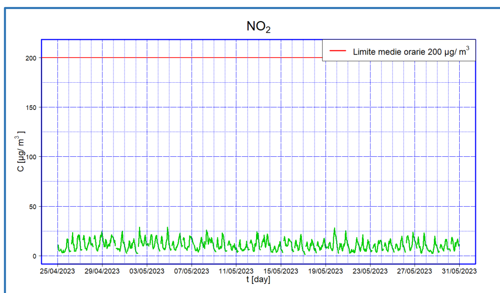
Figura 12 - Valori medi orari di concentrazione di \text{NO}_2 – I periodo
