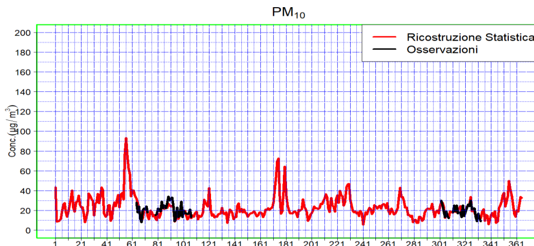
Figura 16: Valori di PM 10 ( \mu\text{g}/\text{m}^3 ) ricostruiti nel 2021 in rosso, mentre in nero i valori osservati
