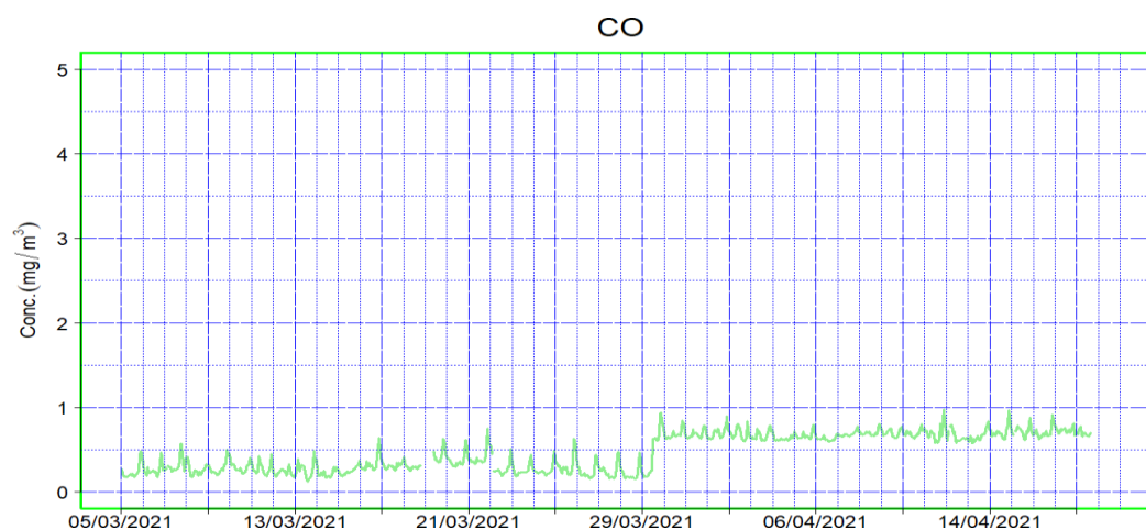
Figura 10: Valori orari di CO nel periodo suddetto (1° campagna)
