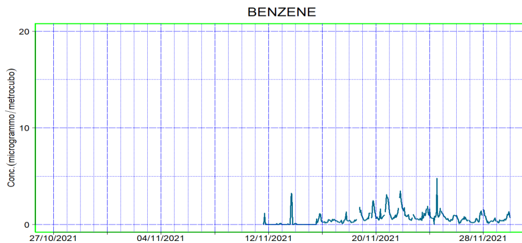
Figura 10: Valori orari di Benzene nel periodo suddetto (II° campagna)
