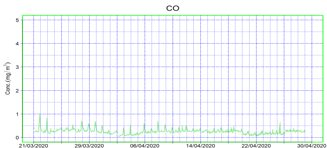
Figura 13: Valori orari di CO nel periodo suddetto (2° campagna)
