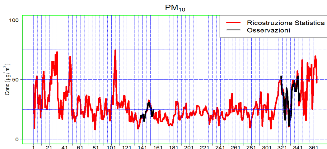
Figura 14: Valori di PM 10 ( \mu\text{g}/\text{m}^3 ) ricostruiti nel 2018 in rosso, mentre in nero i valori osservati
