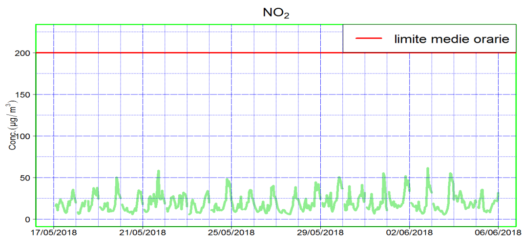
Figura 6: Valori orari di NO 2 nel periodo suddetto (I° campagna)
