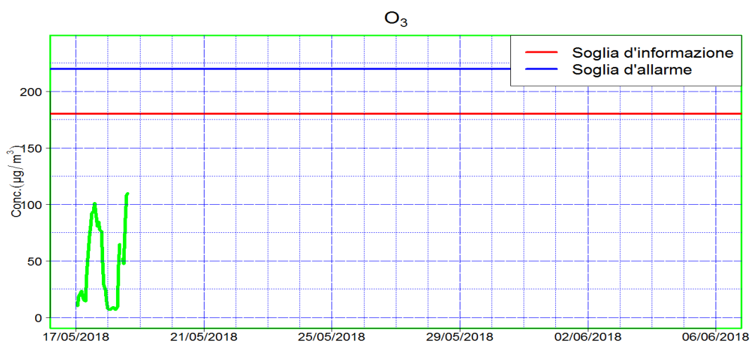
Figura 8: Valori orari di O 3 nel periodo suddetto (I° campagna)
