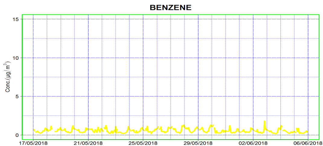
Figura 12: Valori orari di Benzene nel periodo suddetto (I° campagna)
