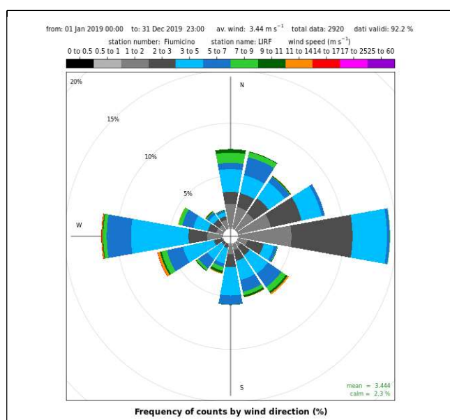
Figura 3.3 - Rosa dei venti di Fiumicino (16242 – LIRF) anno 2019.
