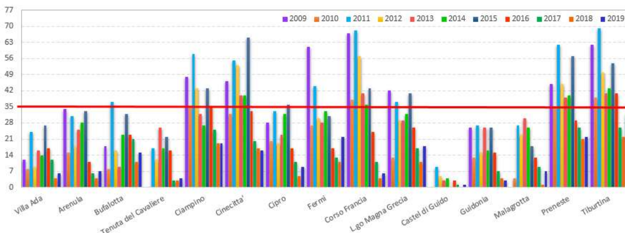
Figura 5.2 - Numero di superamenti del valore limite giornaliero di PM 10 .
