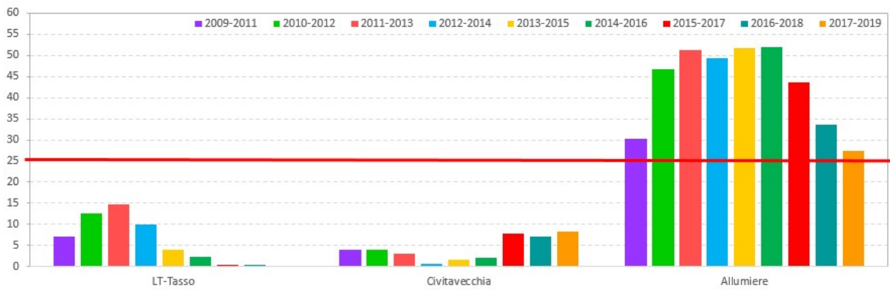
Figura 5.11 - Numero di superamenti di 120 µg/m³ per l'O 3 (mediato su 3 anni).
