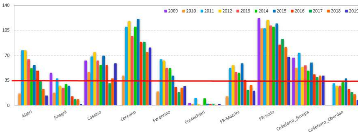
Figura 5.7 - Numero di superamenti del valore limite giornaliero di PM10.
