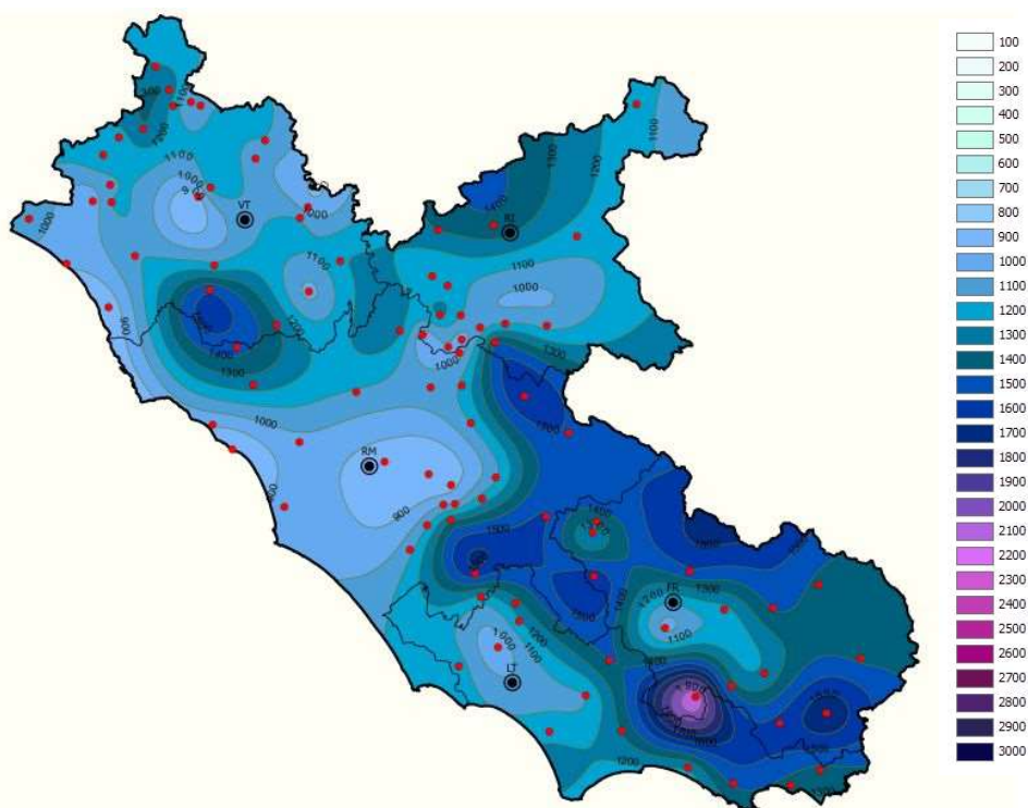
Figura 3.7 - Mappa ARSIAL precipitazioni 2019.
