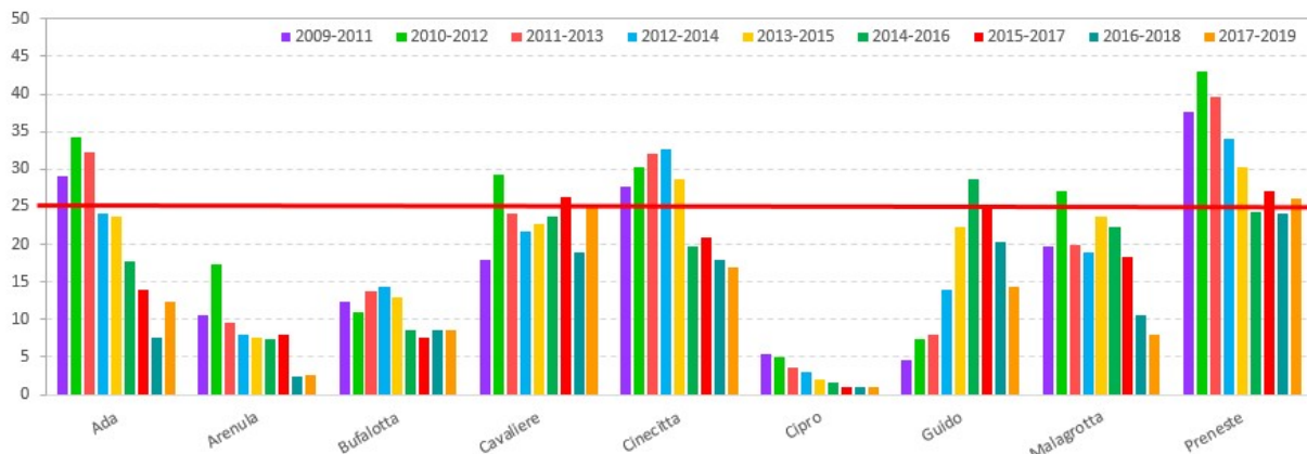
Figura 5.3 - Numero di superamenti di 120 \mu\text{g}/\text{m}^3 per l'O 3 (mediato su 3 anni).
