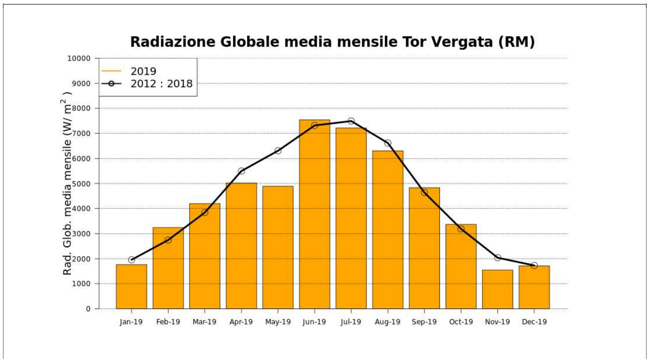
Figura 3.6 - Radiazione globale media mensile 2019 (istogramma) e media climatologica 2012-2018.
