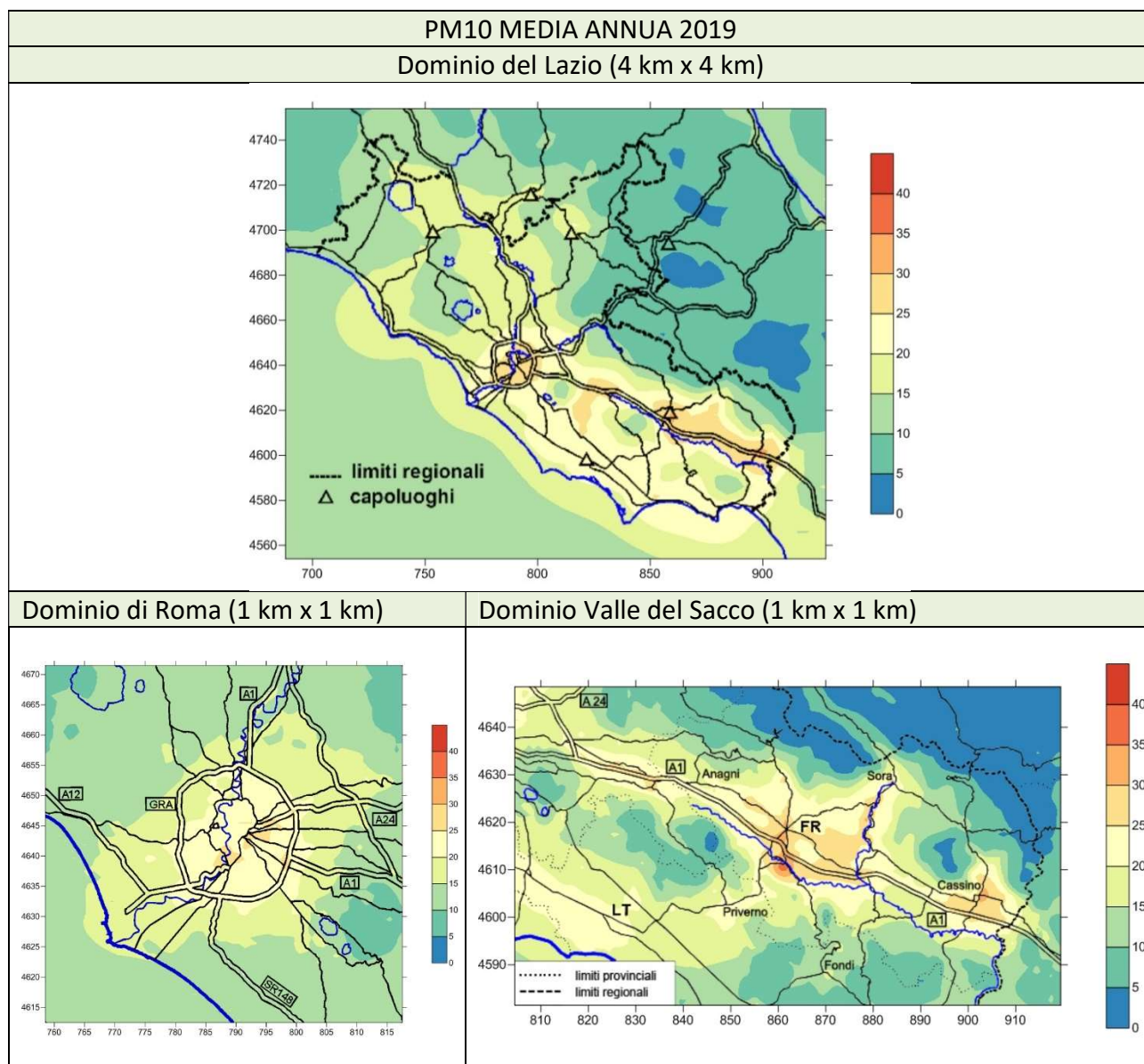
Figura 7.1 - Distribuzione spaziale della media annua di PM10 nel 2019.
