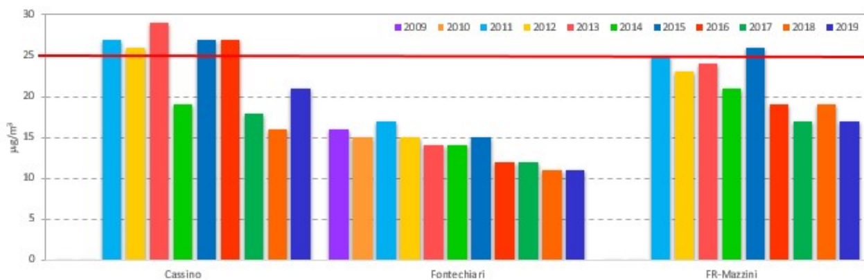
Figura 5.5 - Media annua in \mu\text{g}/\text{m}^3 di PM2.5.
