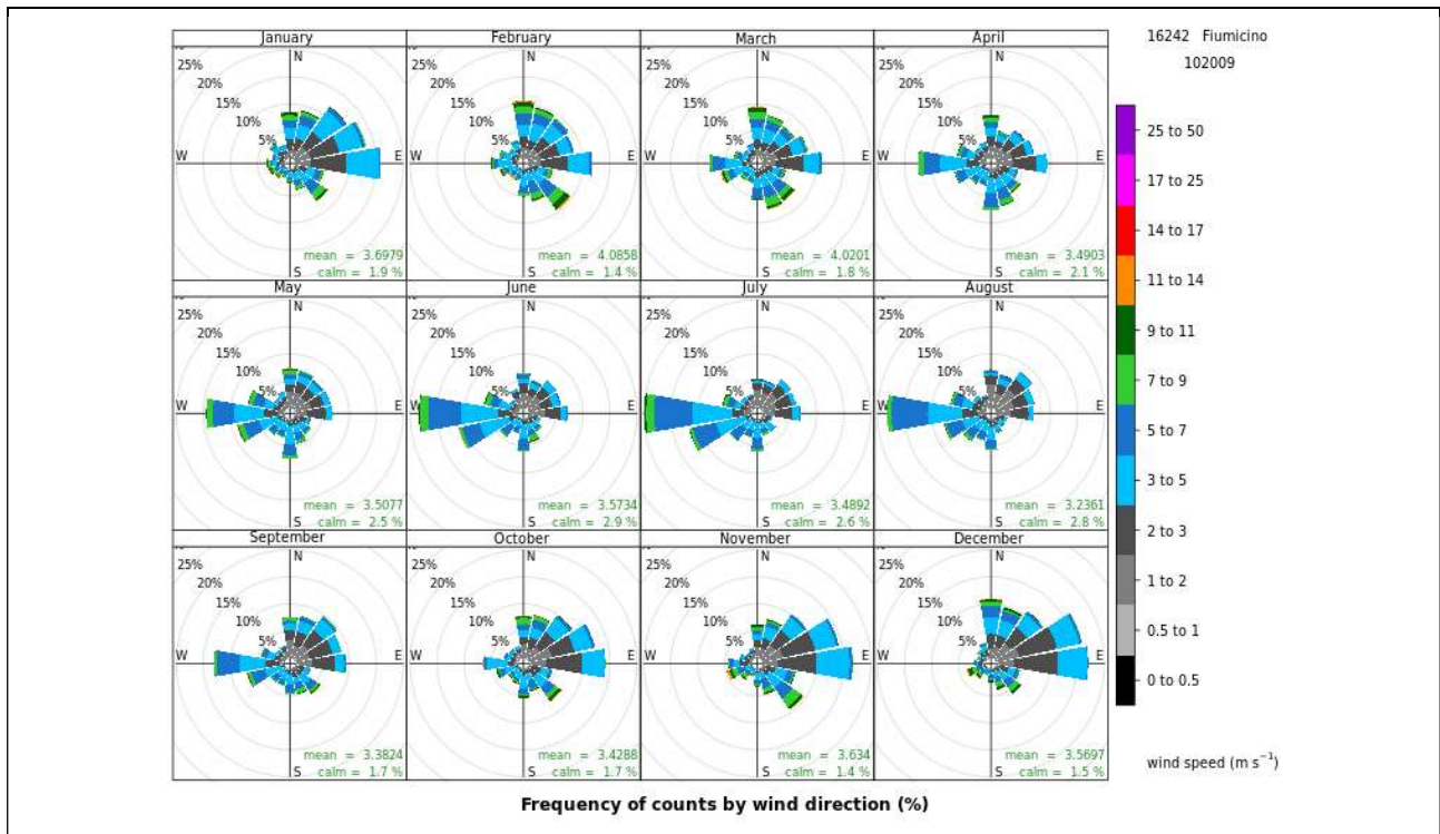
Figura 3.5 - Rosa dei venti di Fiumicino (16242 – LIRF) suddivise per mese.
