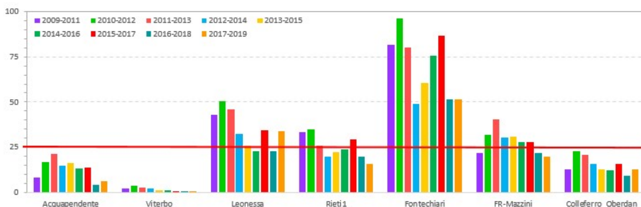
Figura 5.9 - Numero di superamenti di 120 µg/m 3 per l'O 3 (mediato su 3 anni).
