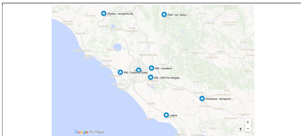
Figura 3.1 - Localizzazione delle stazioni della rete micro-meteorologica.
