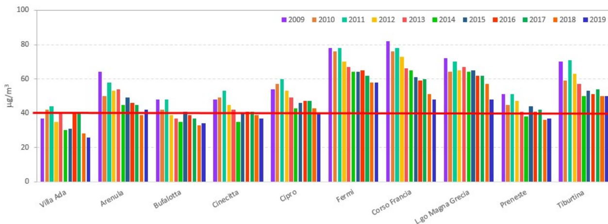
Figura 5.1 - Media Annua NO 2 - stazioni comprese nel GRA di Roma.
