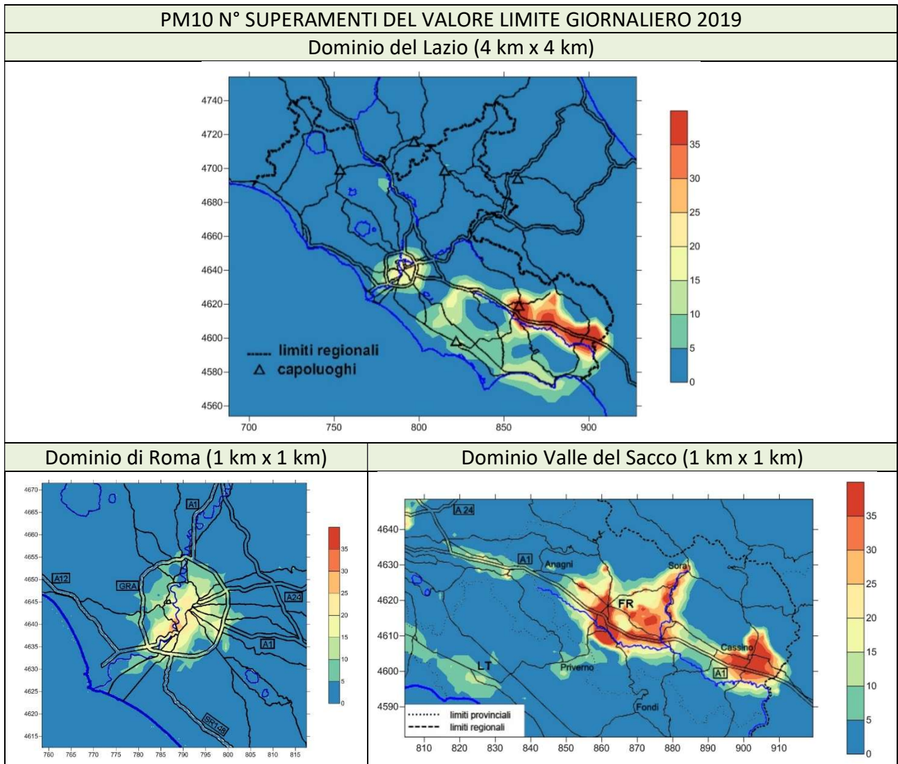
Figura 7.2 - Distribuzione spaziale del numero di superamenti di 50 \mu\text{g}/\text{m}^3 di PM10 nel 2019.
