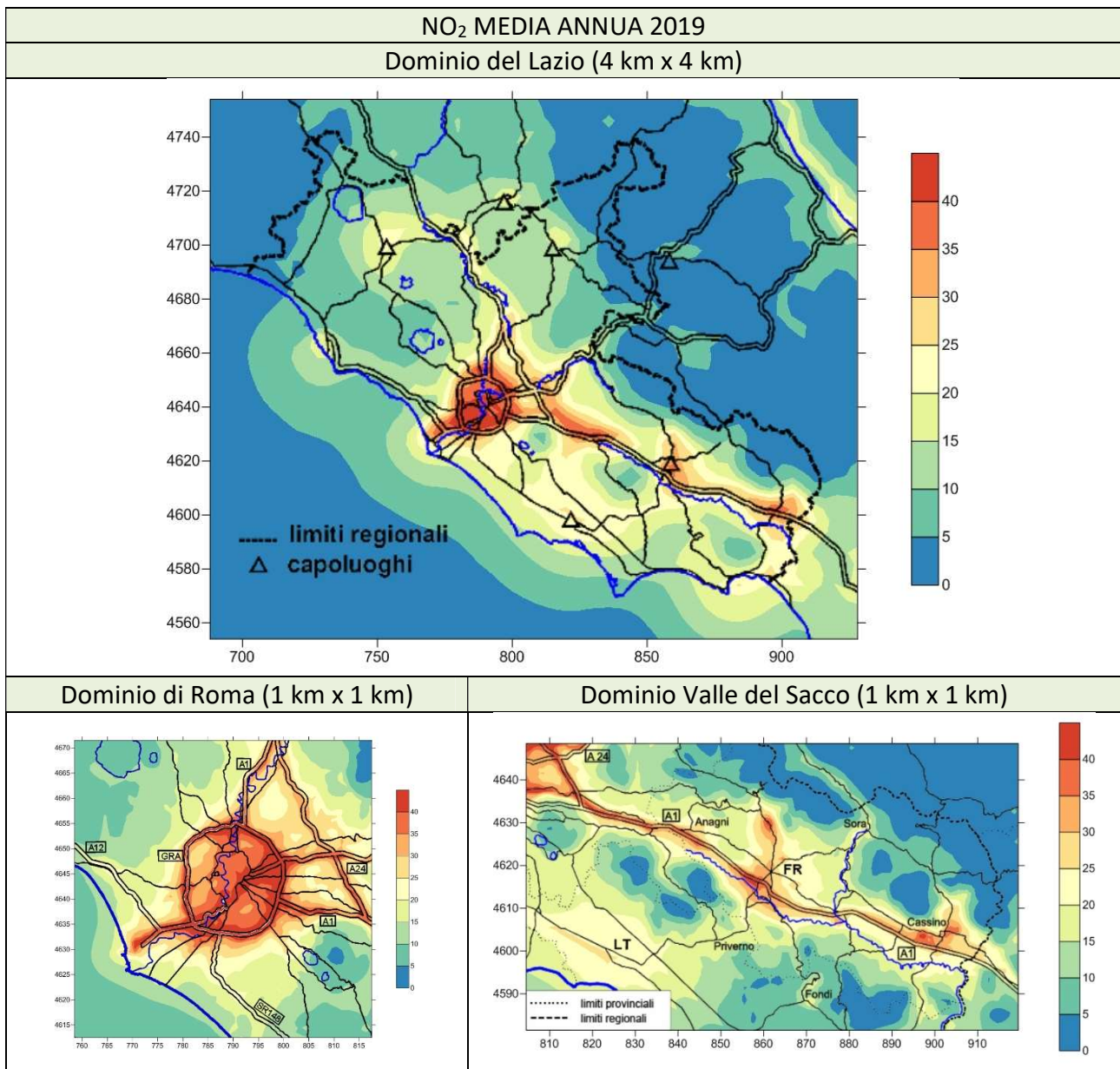
Figura 7.4 - Distribuzione spaziale della media annua di NO 2 nel 2019.
