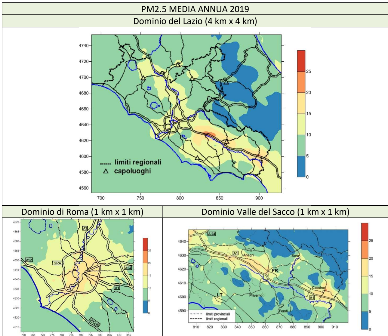
Figura 7.3 - Distribuzione spaziale della media annua di PM2.5 nel 2019.
