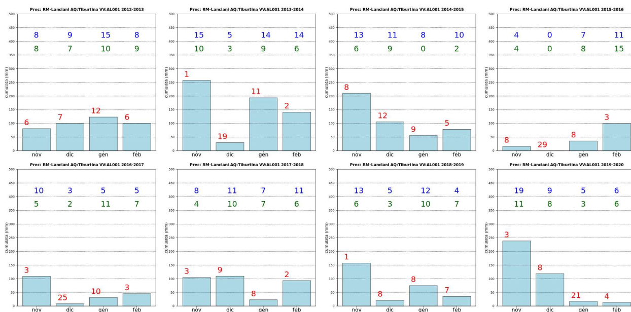
Figura 5.13 - Analisi PM10/parametri meteo stazione Tiburtina.
