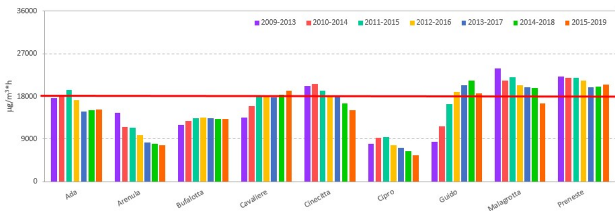
Figura 5.4 - AOT40 per l'O 3 (mediato su 5 anni).
