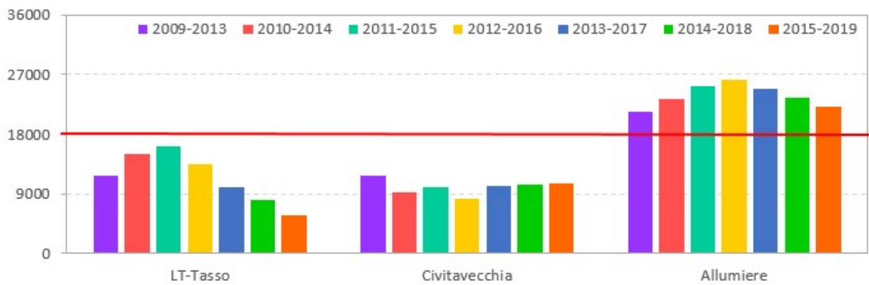
Figura 5.12 - AOT40 per l'O 3 (mediato su 5 anni).
