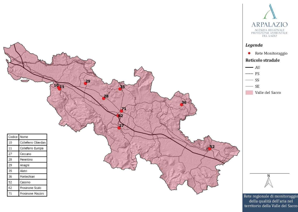
Figura 4.3 - Stazioni di misura nella Valle del Sacco.
