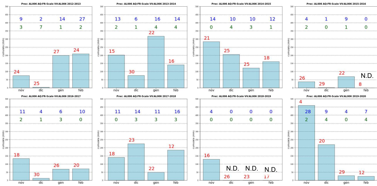
Figura 5.14 - Analisi PM10/parametri meteo stazione Frosinone scalo.
