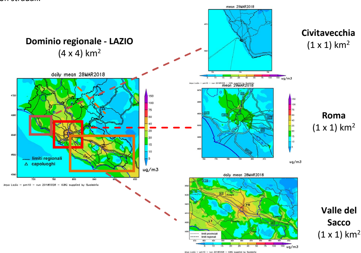
Figura 6.2 - Domini di calcolo del sistema modellistico.
