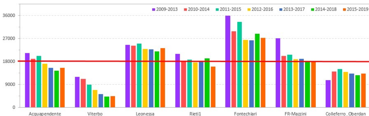
Figura 5.10 - AOT40 per l'O 3 (mediato su 5 anni).
