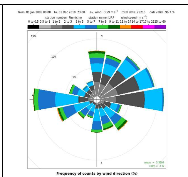
Figura 3.4 - Rosa dei venti di Fiumicino (16242 – LIRF) anni 2009-2018.
