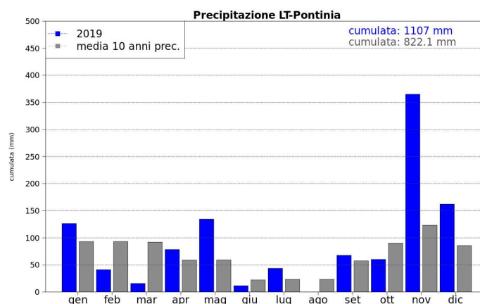
Figura 3.9 - Istogramma mensile della precipitazione cumulata.
