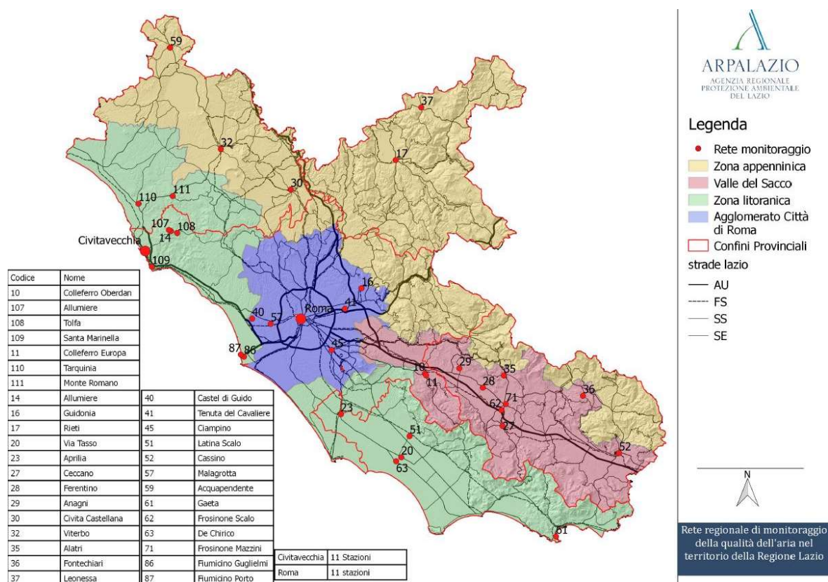
Figura 4.1 - Localizzazione delle stazioni della rete di misura regionale del Lazio nel 2019.
