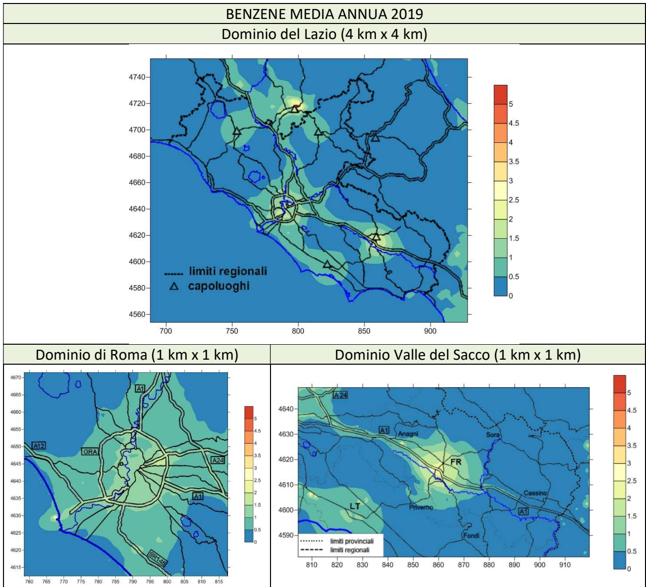
Figura 7.6 - Distribuzione spaziale della media annua di Benzene nel 2019.
