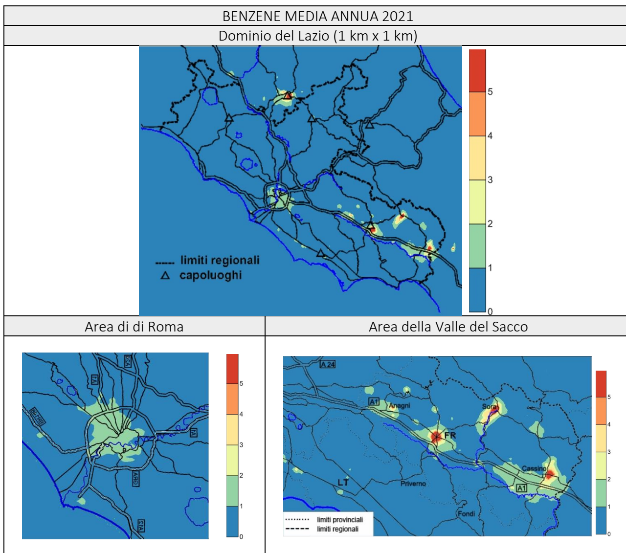
Figura 7.6 - Distribuzione spaziale della media annua di Benzene nel 2021.
