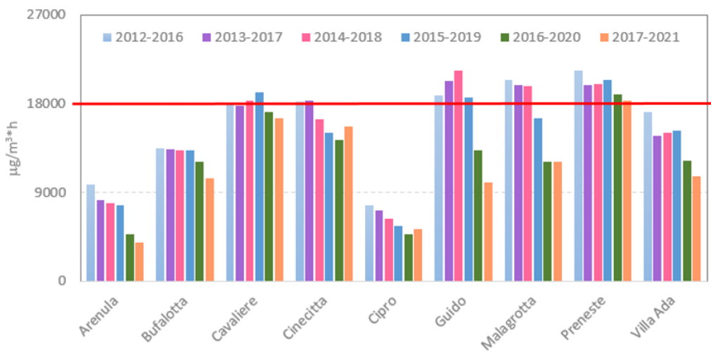
Figura 5.4 - AOT40 per l'O₃ (mediato su 5 anni).
