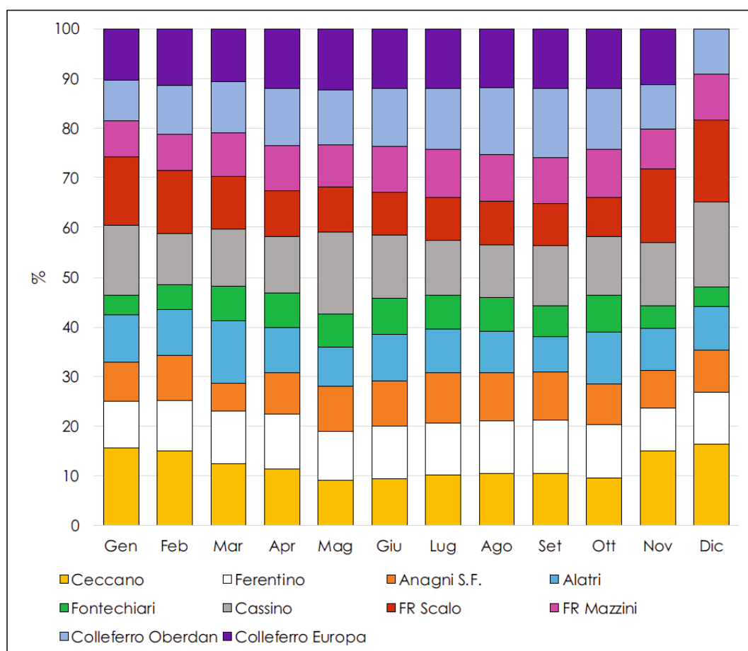
Figura 17. Andamento mensile del contributo percentuale di ciascuna centralina alla concentrazione di PM_{10} nella Valle del Sacco
