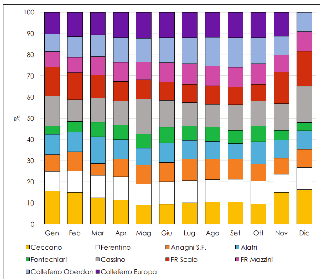
Figura 18. Andamento mensile del contributo percentuale di ciascuna centralina al numero di superamenti del valore limite giornaliero di PM_{10} nella Valle del Sacco
