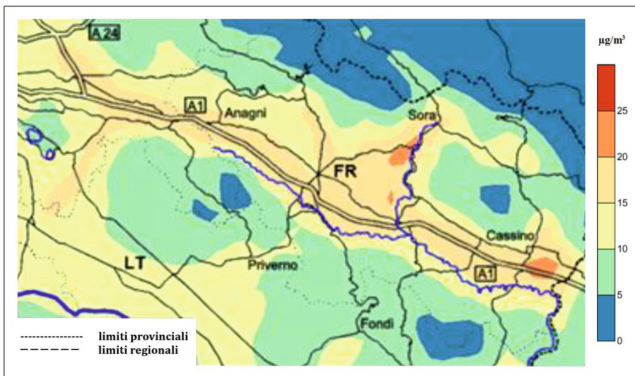
Figura 27. Distribuzione spaziale della media annua di PM_{2.5} nel 2024
