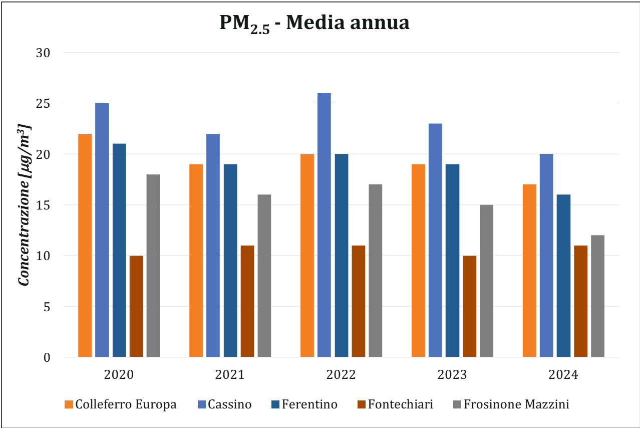
Figura 23. Media annua del PM 2.5 di ciascuna centralina per anno
