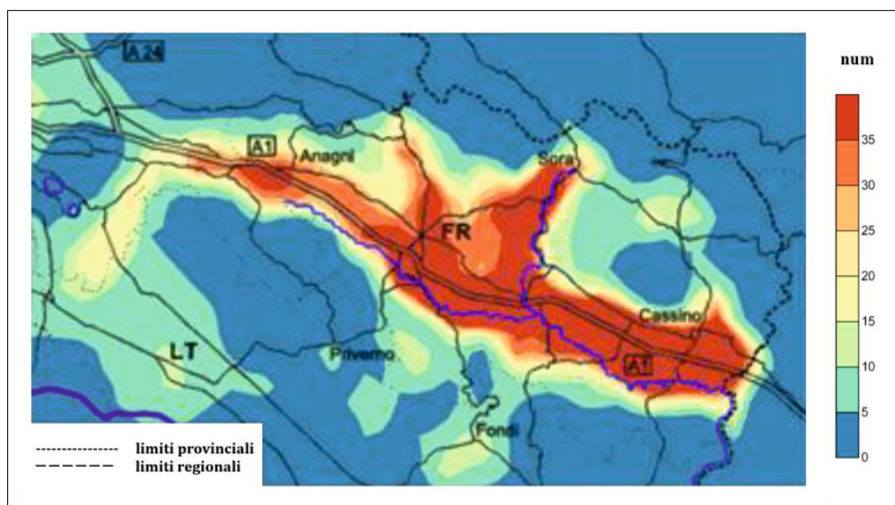
Figura 26. Distribuzione spaziale del numero di superamenti di 50 \mu g/m^3 di PM_{10} nel 2024
