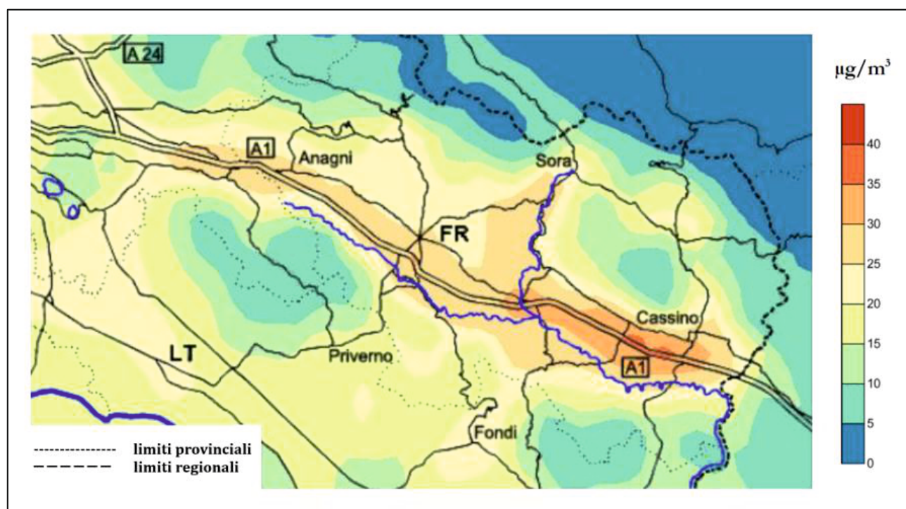
Figura 25. Distribuzione spaziale della media annua di PM_{10} nel 2024
