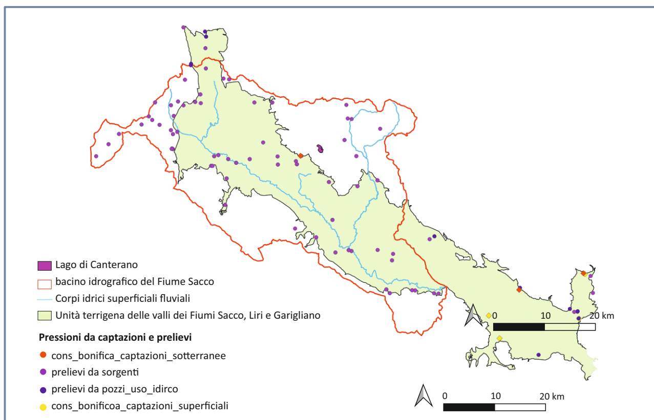
Figura 15. Pressioni puntuali da presenza di siti contaminati e da discariche su corpi idrico lacustre e sotterraneo e su corpi idrici fluviali (in alto). Pressioni puntuali da prelievi per captazioni da corpi idrici superficiali e sotterranei (in basso). Fonte https://sira.arpalazio.it/
