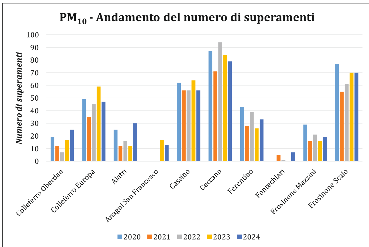
Figura 20. Andamento dei superamenti del PM 10 di ciascuna centralina per anno
