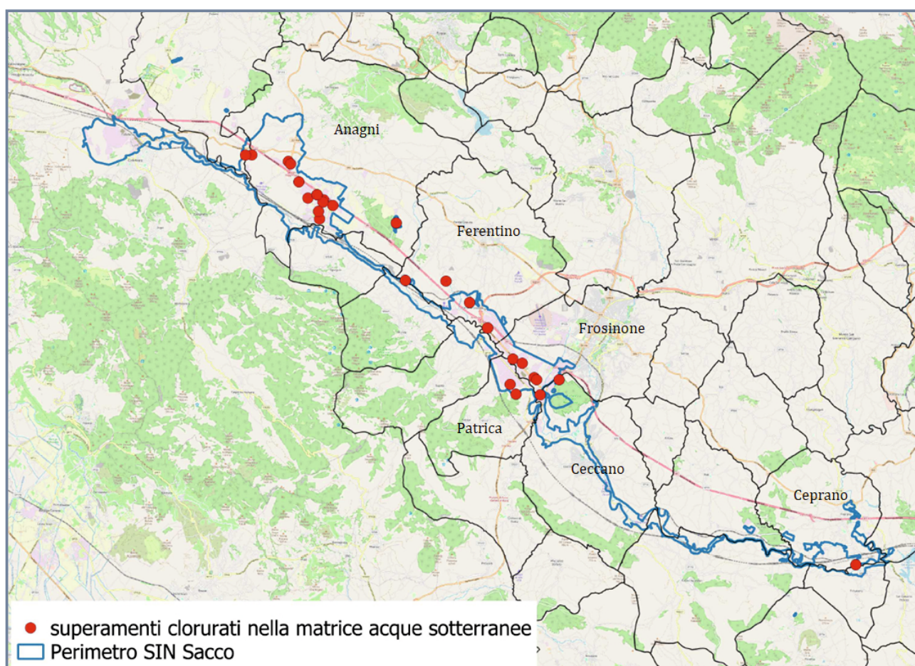
Figura 36. Distribuzione delle contaminazioni da solventi clorurati nelle acque sotterranee
