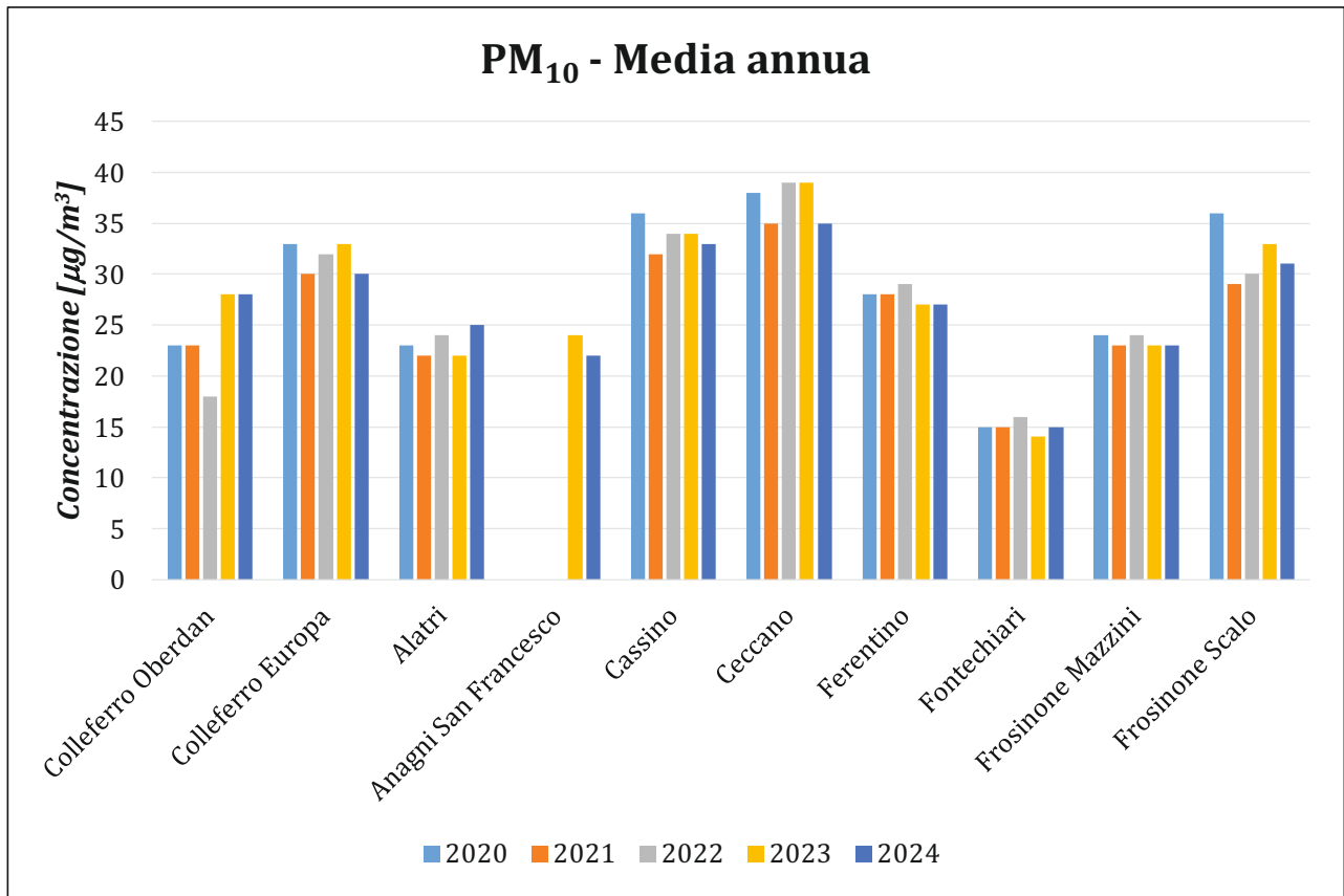
Figura 22. Andamento della media annua del PM 10 di ciascuna centralina per anno
