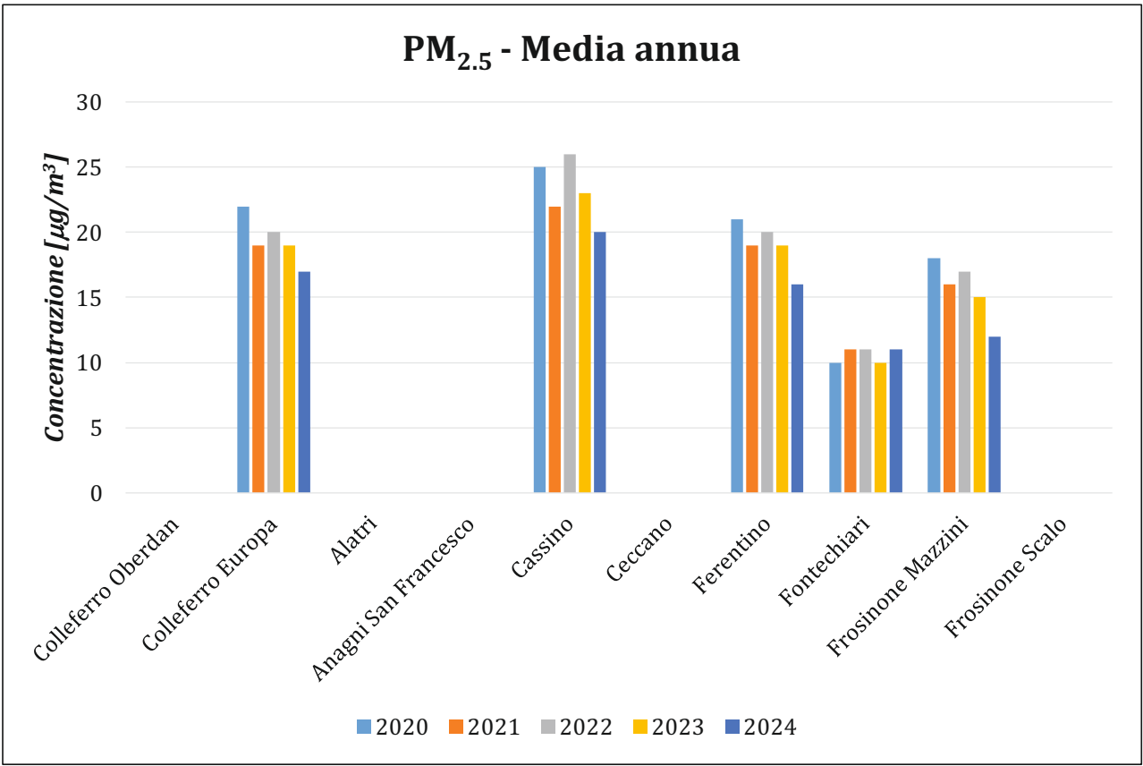
Figura 24. Andamento della media annua del PM 2.5 di ciascuna centralina per anno
