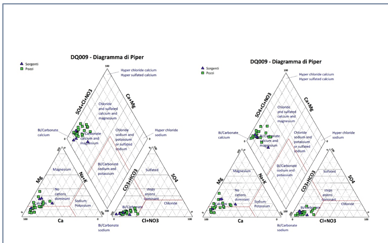
Figura 12. Diagramma di Piper DQ009. A sx dati 1° semestre e a dx dati 2° semestre (dati 2022)
