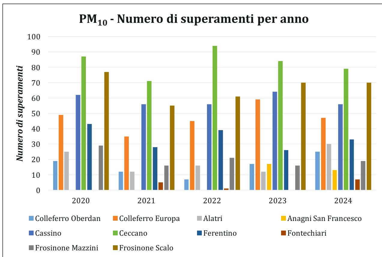
Figura 19. Numero di superamenti del PM 10 di ciascuna centralina per anno
