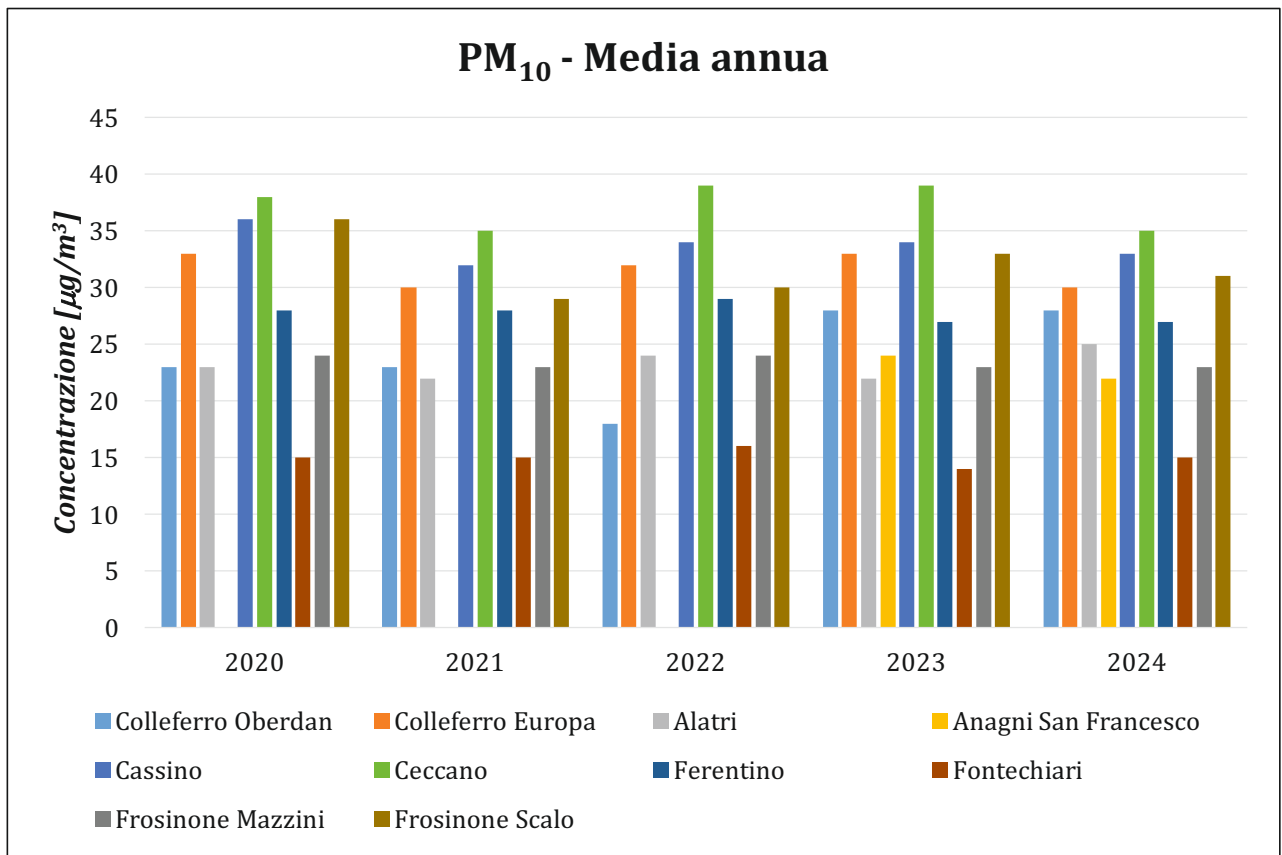
Figura 21. Media annua del PM 10 di ciascuna centralina per anno
